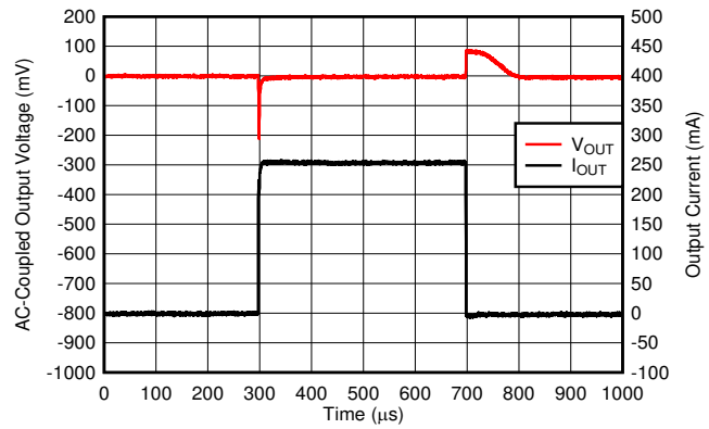
图 6-20. I_{OUT} Transient
