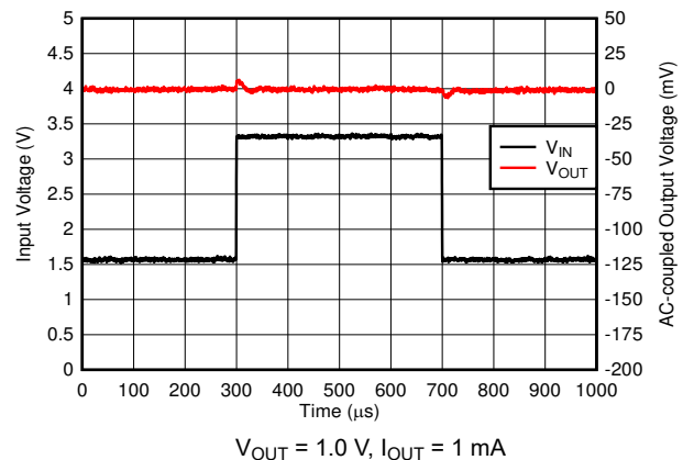
图 6-18. V_{IN} Transient
