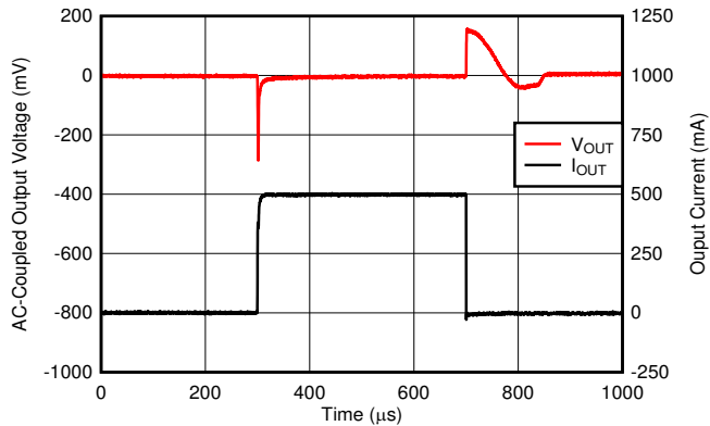
图 6-20. I_{OUT} Transient
