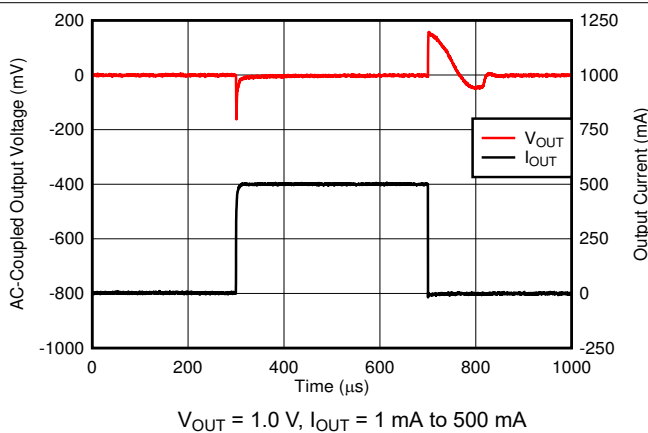
图 6-23. I_{OUT} Transient
