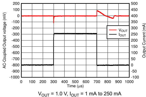
图 6-21. I_{OUT} Transient
