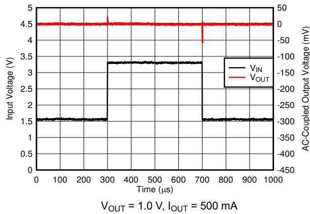
图 6-19. V_{IN} Transient
