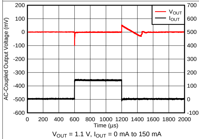
图 9. I_{OUT} Transient
