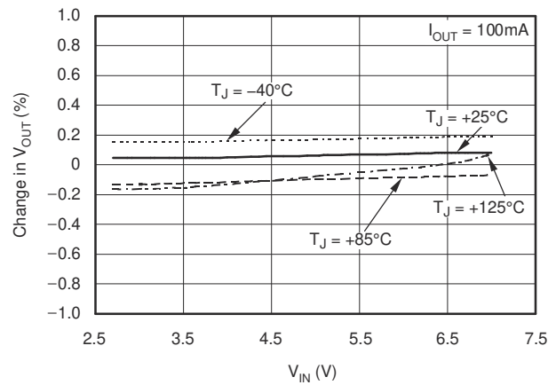
图 6-2. Line Regulation
