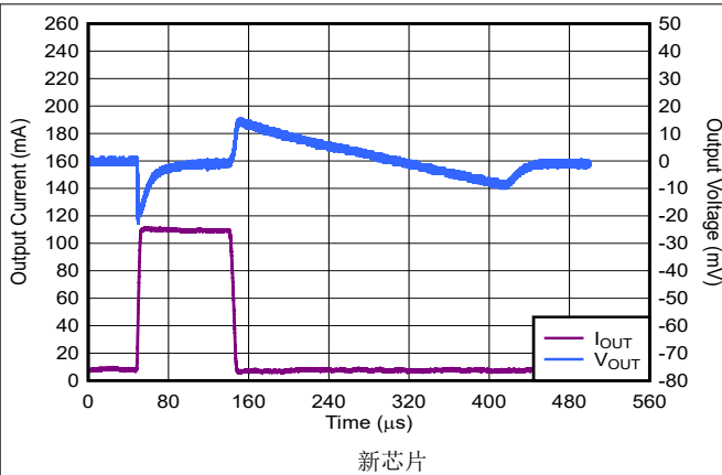
图 5-31. TPS792 负载瞬态响应
