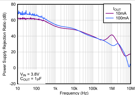
图 5-25. TPS792 波纹抑制与频率
