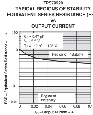
图 5-32. 典型稳定性区域等效串联电阻 (ESR) 与输出电流间的关系
