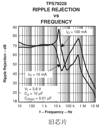
图 5-21. TPS792 波纹抑制与频率
