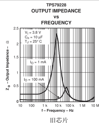
图 5-12. 输出阻抗与频率间的关系
