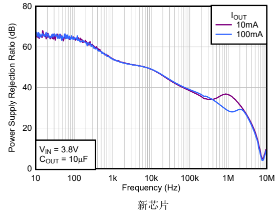
图 5-22. TPS792 波纹抑制与频率
