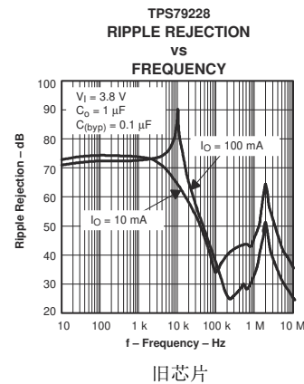
图 5-24. TPS792 波纹抑制与频率
