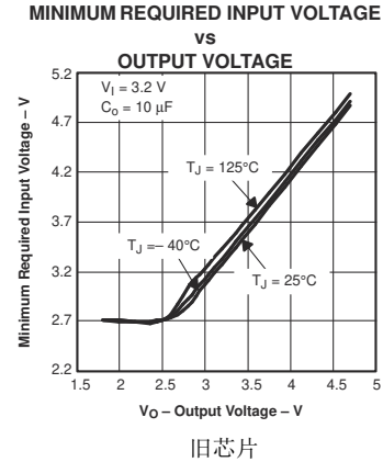
图 5-20. 所需的最小输入电压与输出电压间的关系
