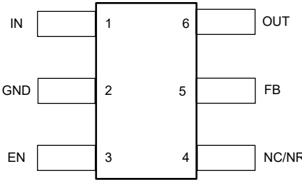
图 4-2. DBV 封装，6 引脚 SOT-23 可调节电压版本（顶视图）
