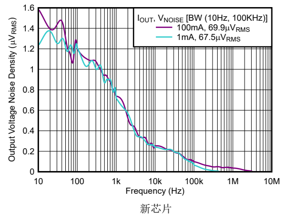
图 5-10. TPS792 输出频谱噪声密度与频率间的关系
