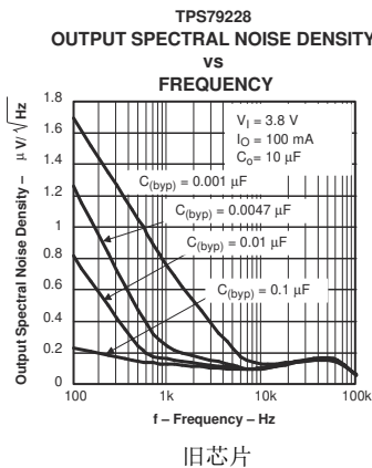
图 5-9. TPS792 输出频谱噪声密度与频率间的关系
