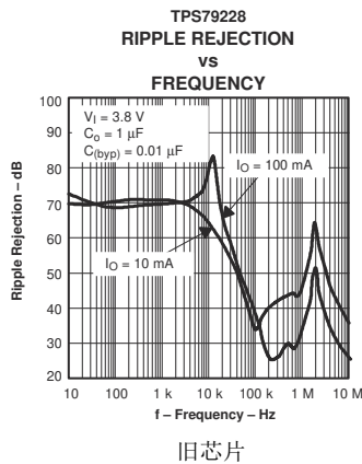
图 5-23. TPS792 波纹抑制与频率
