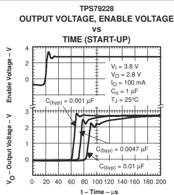
图 5-26. TPS792 输出电压和使能电压与时间之间的关系 (启动)
