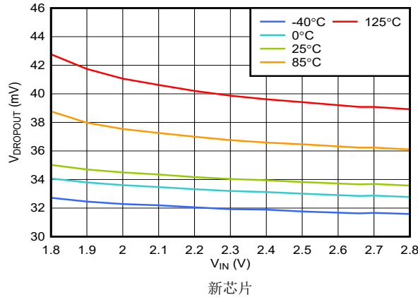
图 5-19. TPS792 压降电压与输入电压间的关系
