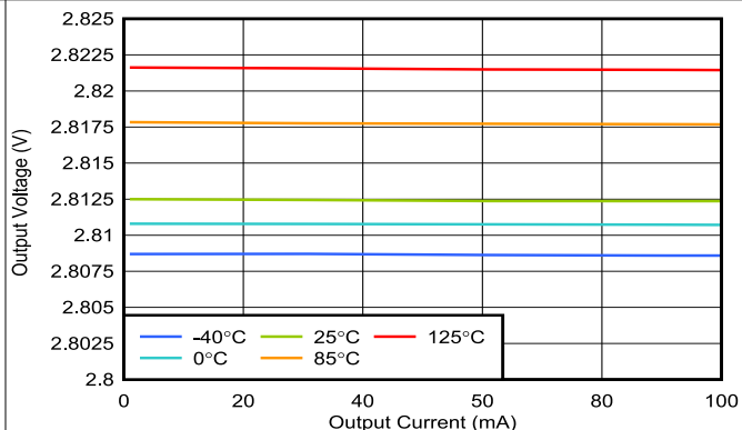
图 5-2. TPS792 输出电压与输出电流间的关系
