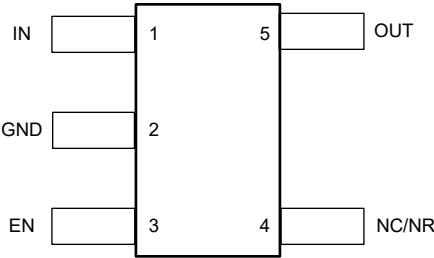
图 4-1. DBV 封装，5 引脚 SOT-23 固定电压版本（顶视图）
