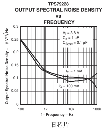
图 5-7. TPS792 输出频谱噪声密度与频率间的关系
