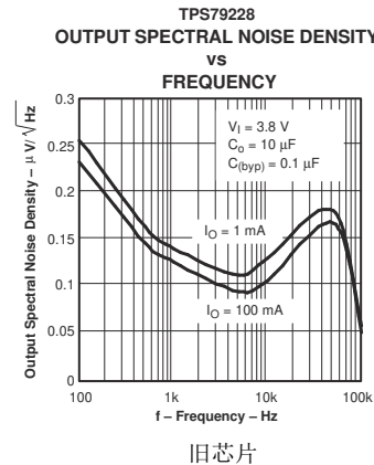
图 5-8. TPS792 输出频谱噪声密度与频率间的关系
