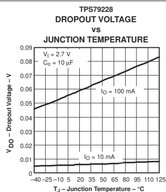
图 5-14. TPS792 压降电压与结温间的关系
