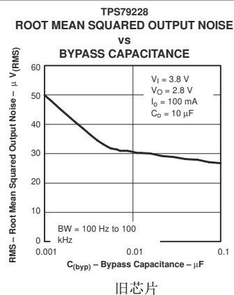
图 5-11. 均方根输出噪声与旁路电容间的关系
