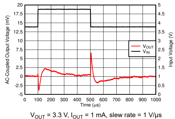
图 6-16. Line Transient
