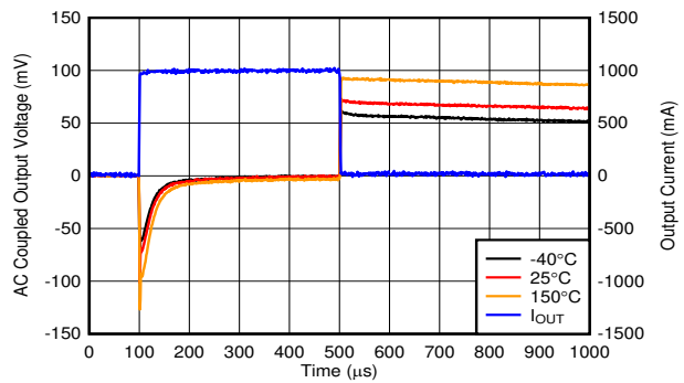
图 6-20. Load Transient vs Temperature
