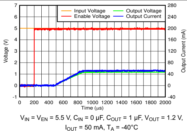
图 6-29. Start Up
