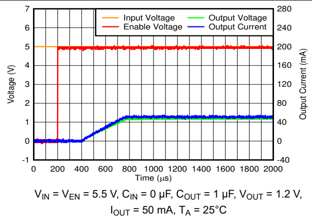
图 6-30. Start Up
