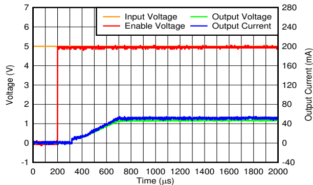
图 6-31. Start Up
