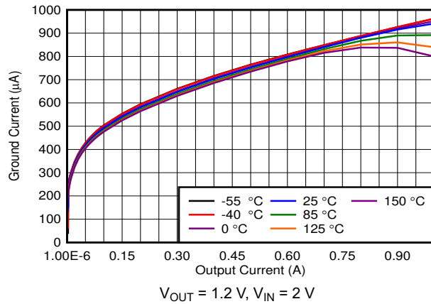
图 6-9. I_{\text{GND}} vs I_{\text{OUT}}
