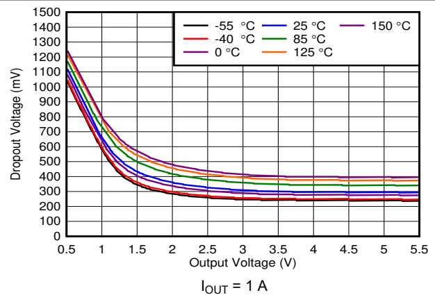
图 6-6. Dropout vs Output Voltage
