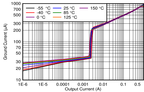
图 6-8. I_{\text{GND}} vs I_{\text{OUT}}
