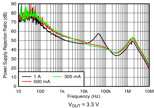
图 6-27. PSRR vs I_{OUT}
