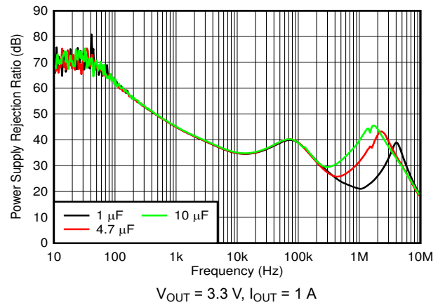
图 6-26. PSRR vs C_{OUT}
