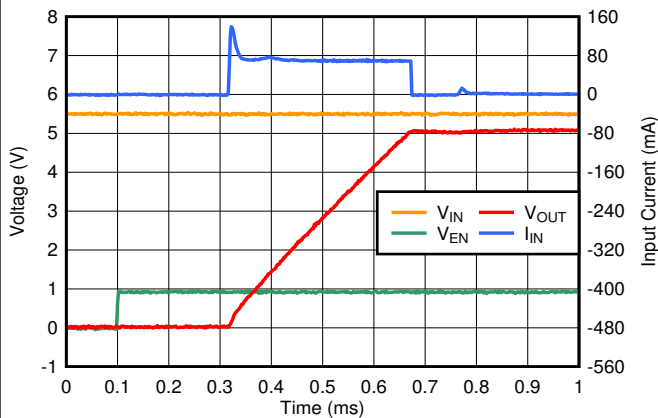
图 6-31. Start Up
