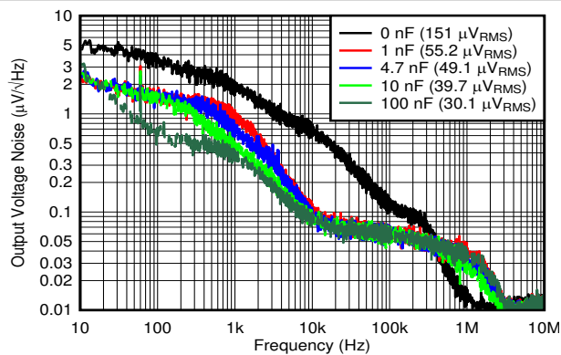
图 6-23. Noise vs C_{FF}
