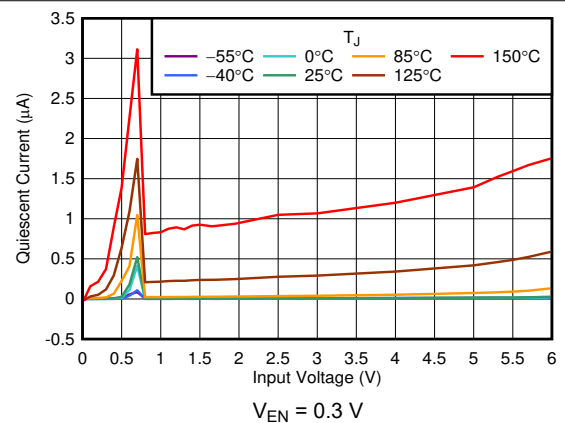
图 6-12. I_{\text{SHDN}} vs V_{\text{IN}}
