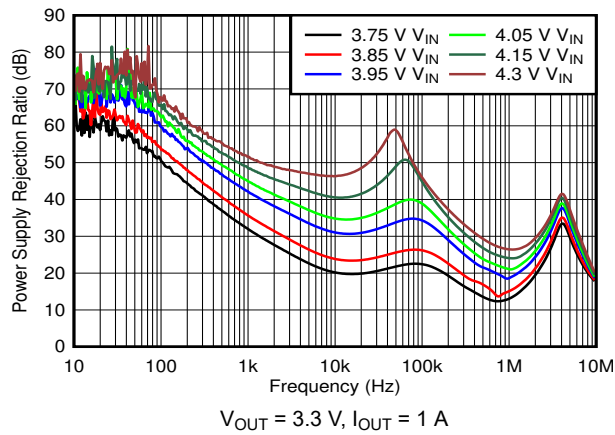
图 6-25. PSRR vs V_{IN}
