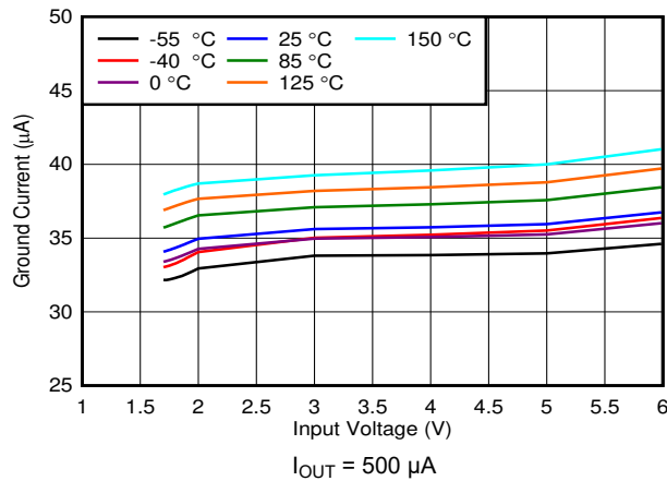
图 6-7. I_{\text{GND}} vs V_{\text{IN}}
