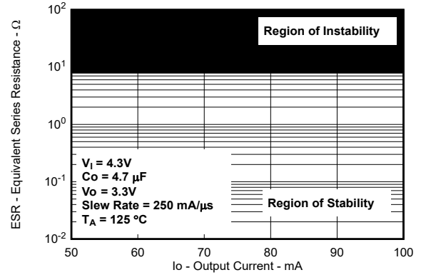
图 5-53. 典型稳定性 ESR 区域与输出电流间的关系（旧芯片）
