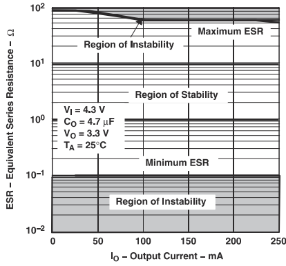
图 5-52. 典型稳定性 ESR 区域与输出电流间的关系（旧芯片）
