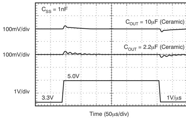
Legacy chip 图 5-32. V_{BIAS} Line Transient
