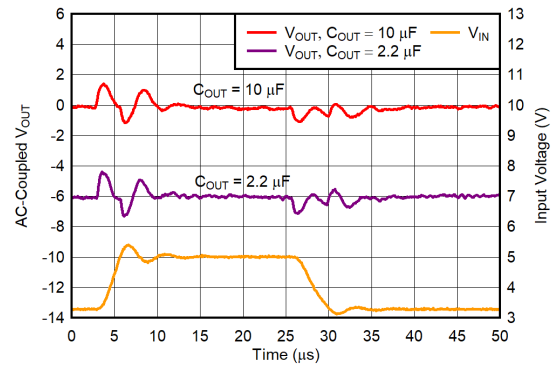
New chip 图 5-33. V_{BIAS} Line Transient
