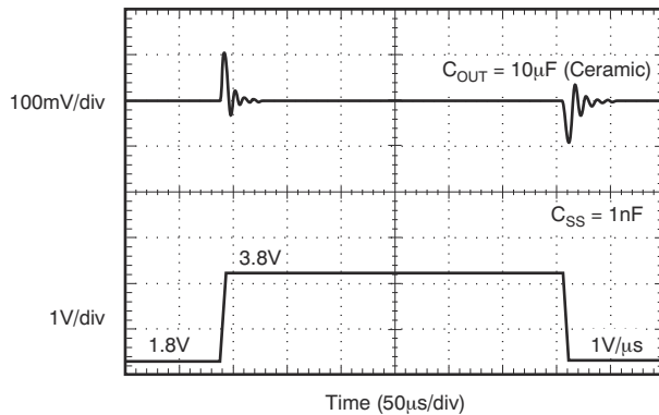
Legacy chip 图 5-32. V_{BIAS} Line Transient
