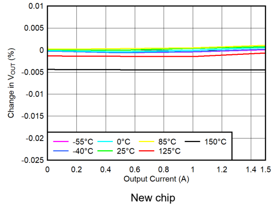
图 5-8. Load Regulation
