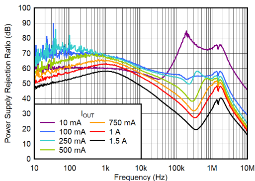
图 5-3. 在 V OUT = 0.8V 时，IN PSRR 与频率和 I OUT 间的关系
