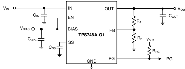
图 7-2. 典型 ADJ 电压应用
