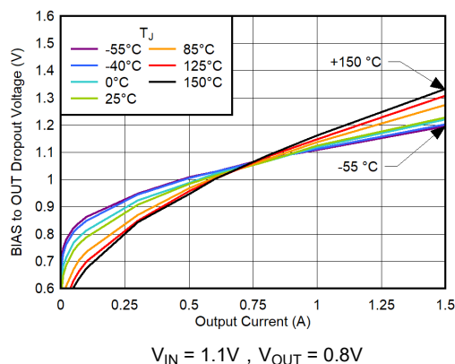
图 5-12. BIAS 至 OUT 压降电压与 I_{OUT} 和温度 ( T_J ) 间的关系
