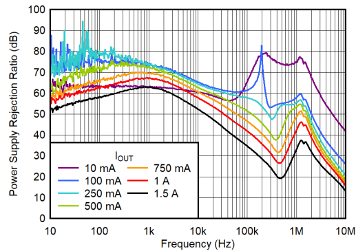
图 7-3. 在 V_{OUT} = 1.8V 时, PSRR 与频率间的关系
