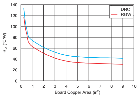
图 7-4. R_{\theta JA} 与电路板尺寸之间的关系
