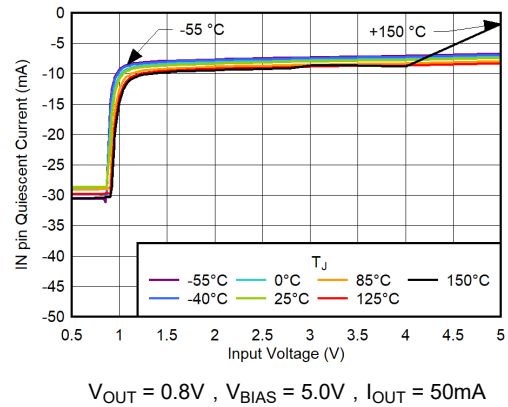
图 5-17. IN 引脚静态电流与输入电压间的关系
