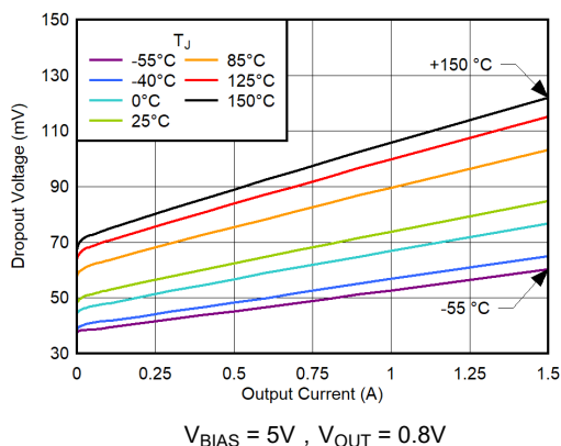
图 5-11. IN 至 OUT 的压降电压与 I_{OUT} 和温度 ( T_J ) 间的关系
