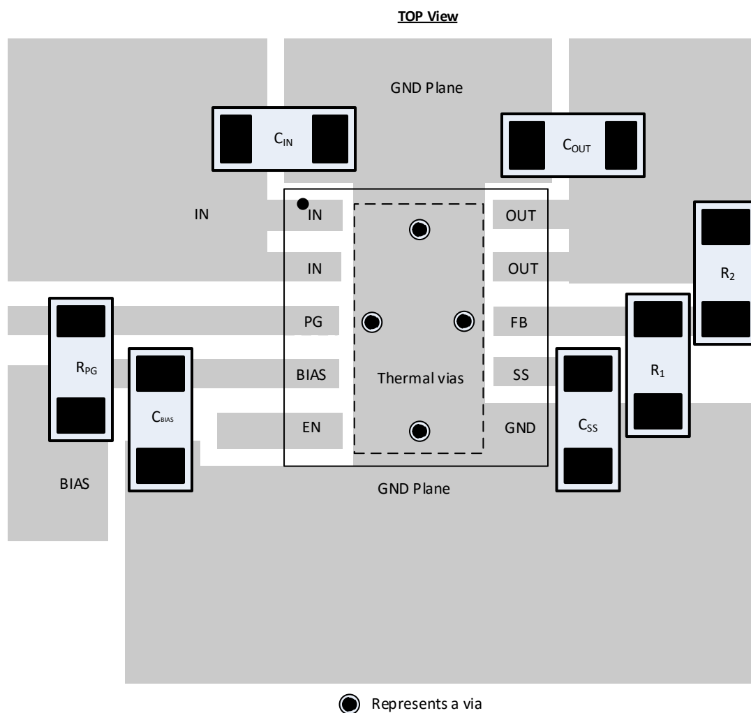
图 7-5. 示例布局
