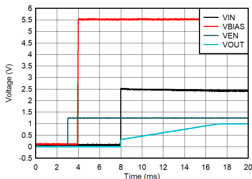
图 7-1. V_{OUT} = 1V 时的时序控制和软启动行为
