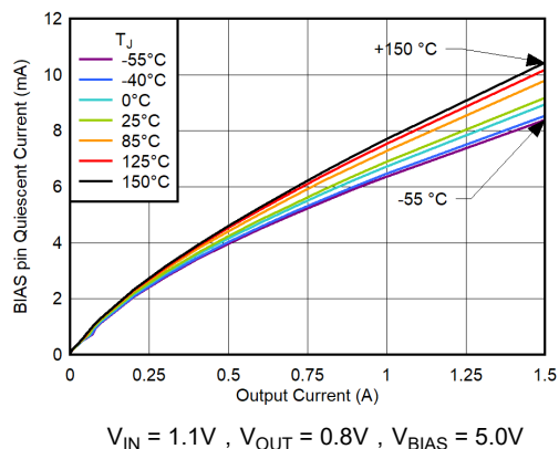
图 5-20. BIAS 引脚静态电流与输出电流间的关系
