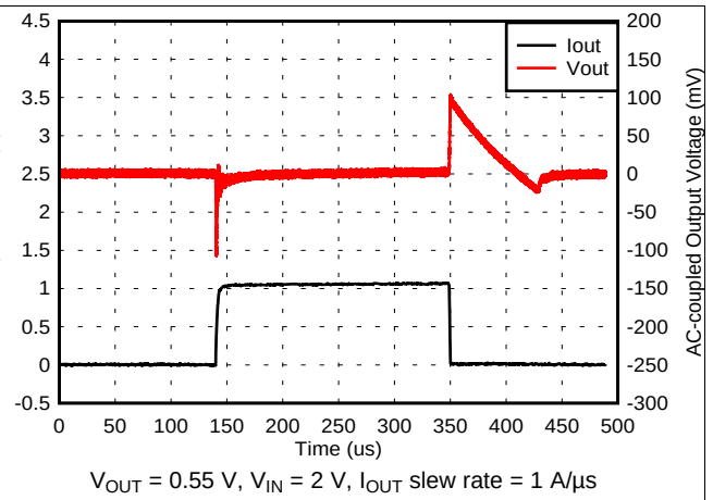
图 26. 1-mA to 1-A Load Transient (0.55 V)
