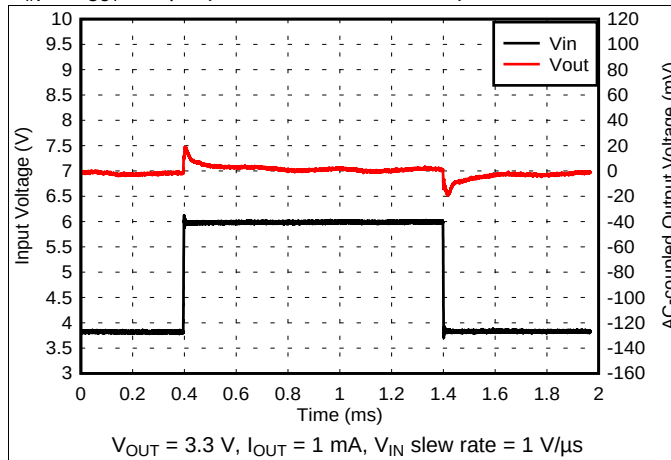
图 25. 3.3-V Line Transient
