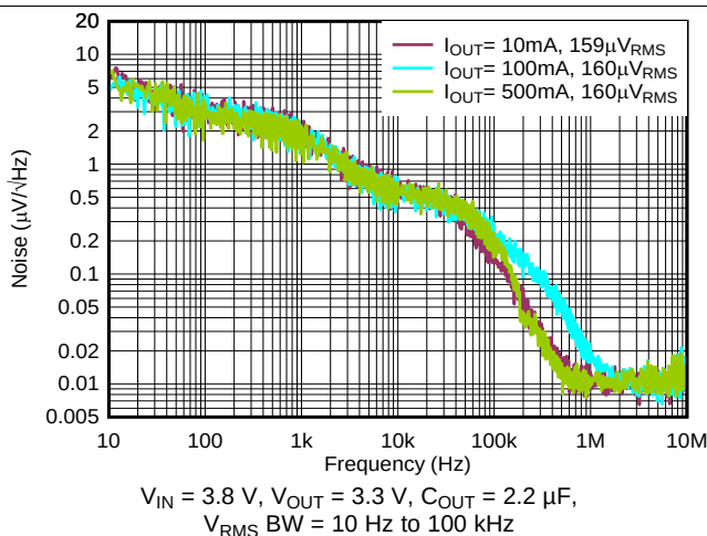
图 41. Output Spectral Noise Density
