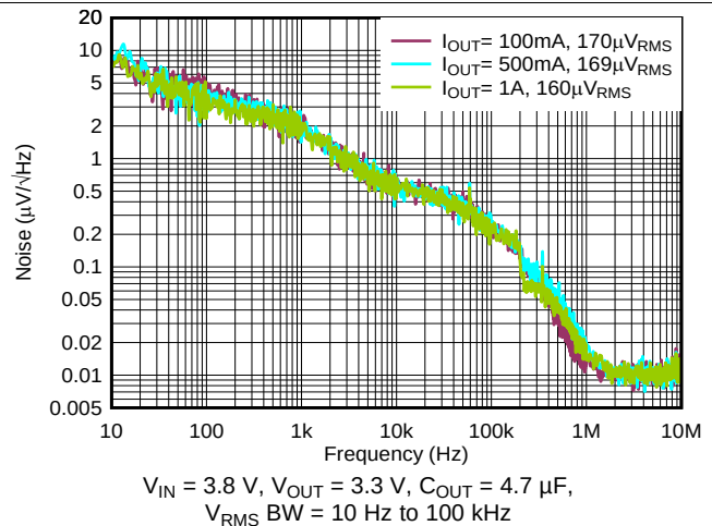
图 40. Output Spectral Noise Density
