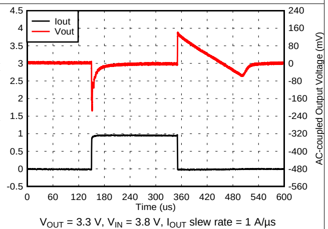
图 28. 1-mA to 1-A Load Transient (3.3 V)
