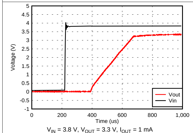
图 29. V_{IN} Power-Up
