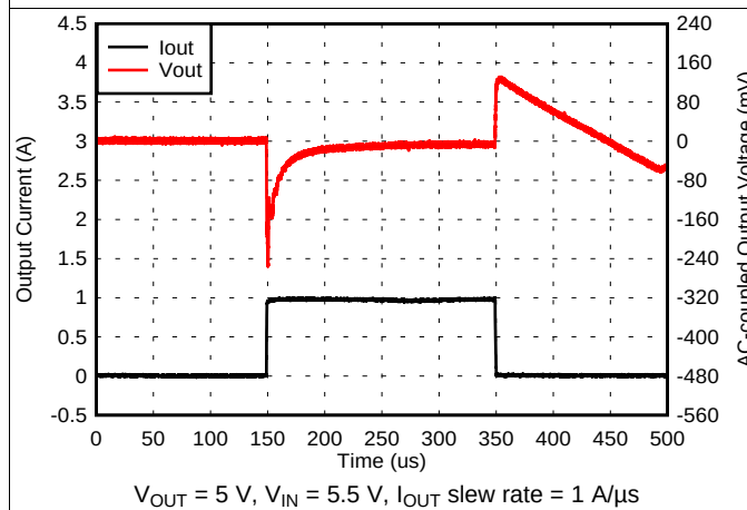
图 27. 1-mA to 1-A Load Transient (5 V)
