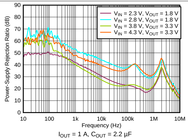
图 36. PSRR vs Frequency
