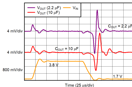
新芯片 图 5-32. V_{IN} 线路瞬态 (新芯片)
