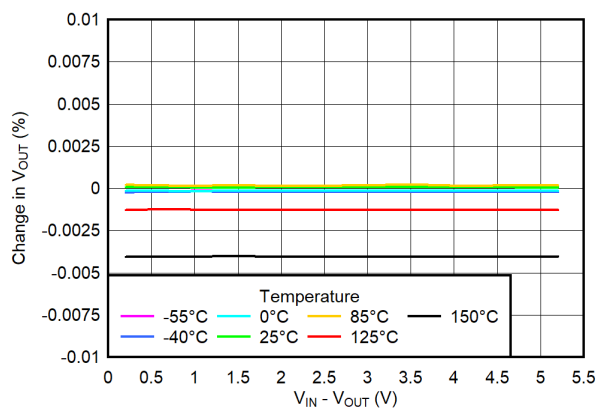
图 5-6. 线路调节 (新芯片)
