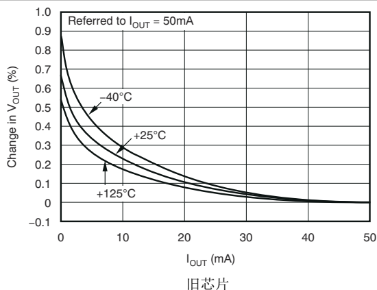
图 5-1. 负载调整率
