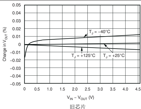
图 5-5. 线性调整率
