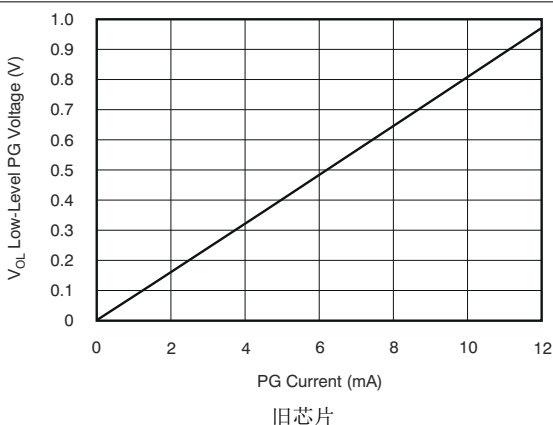
图 5-29. 低电平 PG 电压与 PG 电流间的关系
