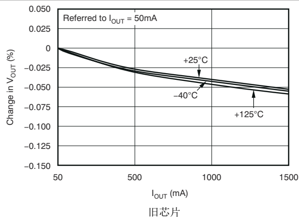
图 5-3. 负载调整率
