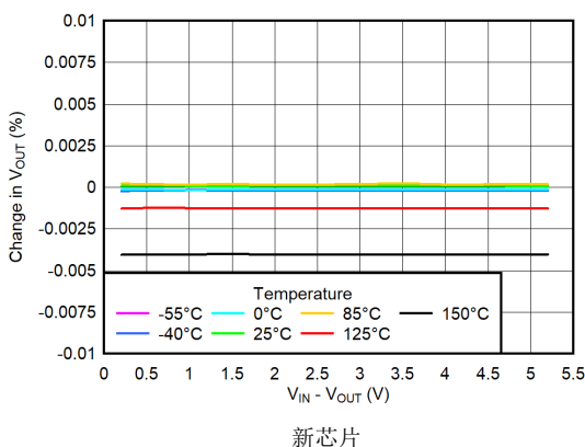
图 5-6. 线性调整率
