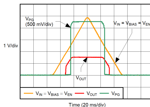
图 5-40. 上电、断电
