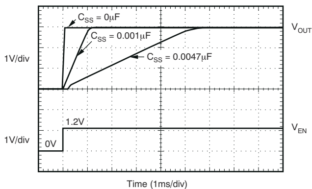
图 5-37. 导通响应
