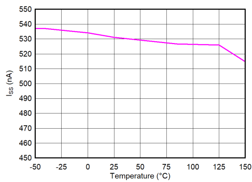
图 5-28. 软启动充电电流 ( I_{\text{SS}} ) 与温度 ( T_J ) 间的关系
