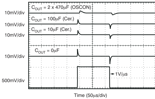
图 5-31. V_{BIAS} 线路瞬态 (1.5A)
