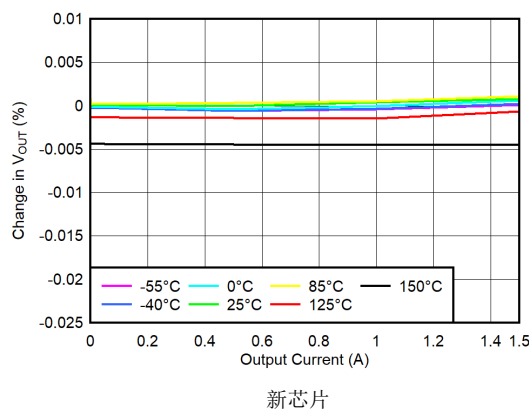
图 5-4. 负载调整率
