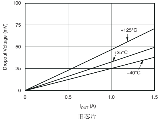
图 5-7. V_{IN} 压降电压与 I_{OUT} 和温度 ( T_J ) 间的关系
