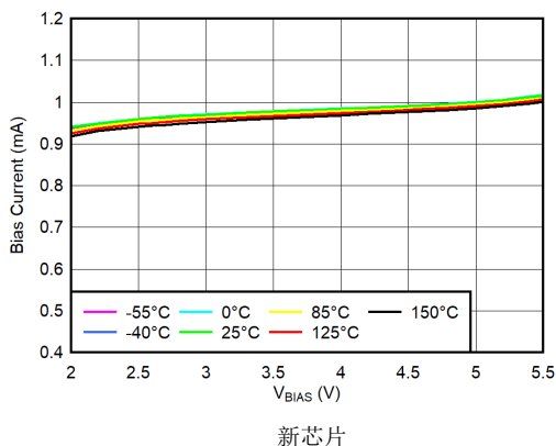
图 5-25. BIAS 引脚电流与 V_{\text{BIAS}} 和温度 ( T_J ) 间的关系
