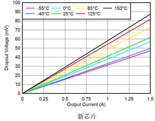
图 5-8. V_{IN} 压降电压与 I_{OUT} 和温度 ( T_J ) 间的关系
