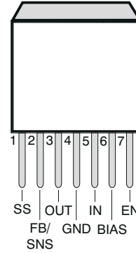
图 4-2. KTW 封装，7 引脚 DDPak/TO-263（顶视图，旧芯片）
