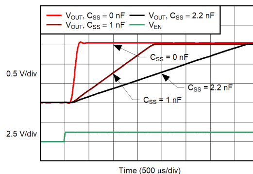
图 5-38. 导通响应
