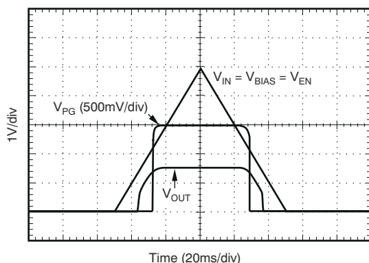
图 5-37. 导通响应
