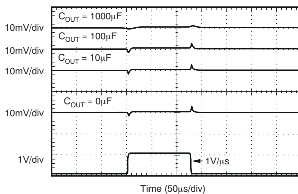
图 7-6. V_{BIAS} 线路瞬态 ( 1.5A )
