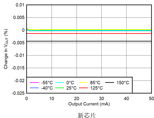
图 5-2. 轻负载下的负载调整率
