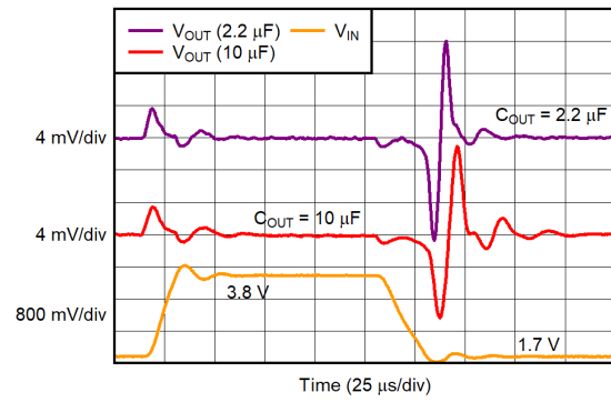
图 5-34. V_{IN} 线路瞬态
