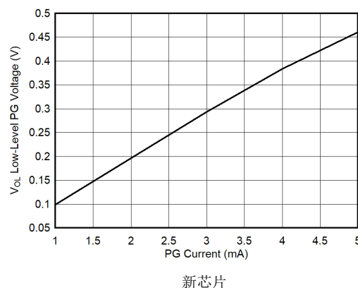
图 5-30. 低电平 PG 电压与电流间的关系
