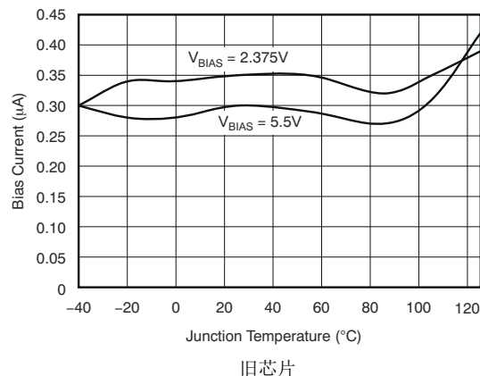
图 5-26. I_{\text{BIAS}} 关断与温度间的关系
