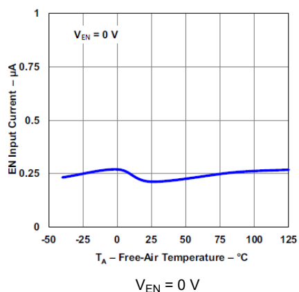
图 5-9. EN Input Current vs Temperature
