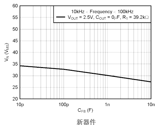
图 5-30. TPS73701-Q1 RMS 噪声电压与 C_{FB} 间的关系
