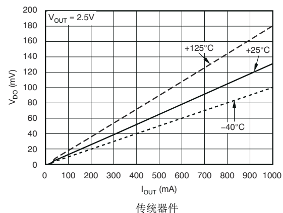
图 5-5. 压降电压与输出电流间的关系
