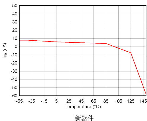
图 5-48. TPS73701-Q1 I_{FB} 与温度间的关系
