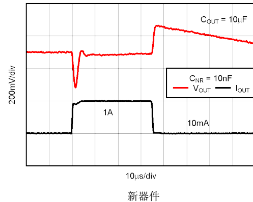
图 5-36. TPS73733-Q1 负载瞬态响应
