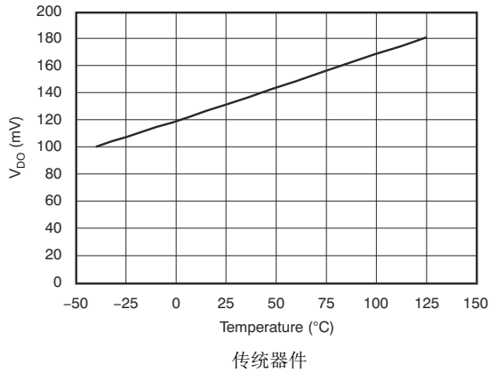
图 5-7. 压降电压与温度间的关系
