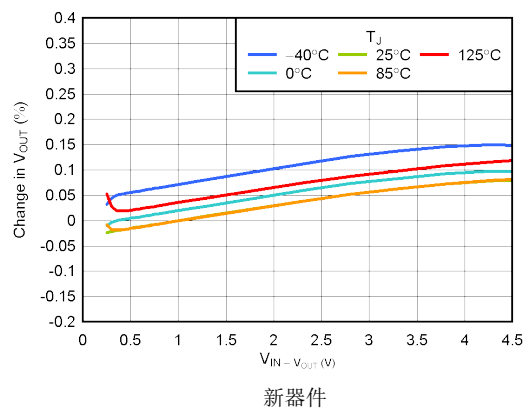
图 5-4. 线性调整率
