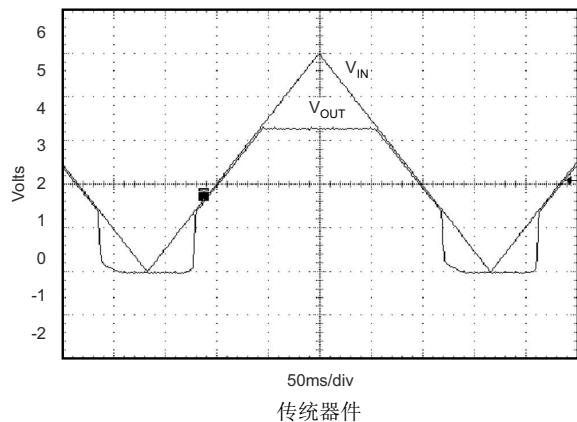
图 5-43. TPS73701-Q1、 V_{OUT} = 3.3\text{V} 上电和断电
