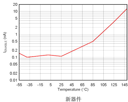
图 5-46. I_{EN} 与温度间的关系
