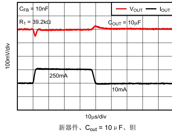
图 5-50. TPS73701-Q1 负载瞬态, 可调节版本
