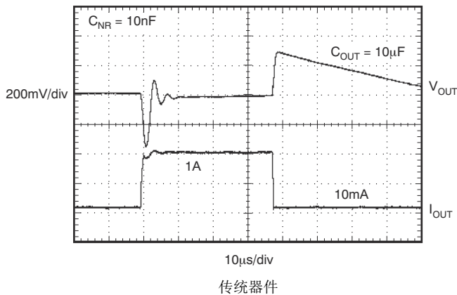
图 5-35. TPS73733-Q1 负载瞬态响应
