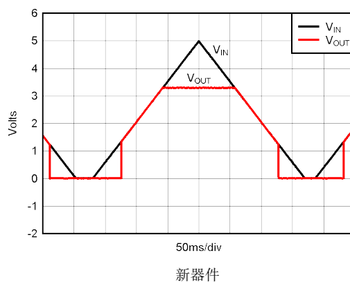
图 5-44. TPS73701-Q1、 V_{OUT} = 3.3\text{V} 上电和断电
