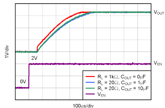
图 7-4. TPS737-Q1 导通响应
