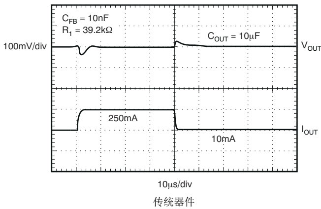
图 5-49. TPS73701-Q1 负载瞬态, 可调节版本
