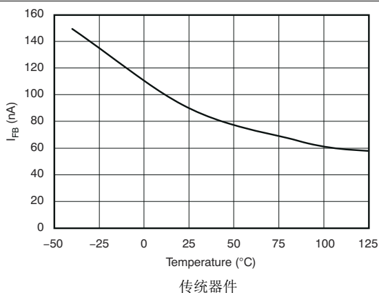
图 5-47. TPS73701-Q1 I_{FB} 与温度间的关系
