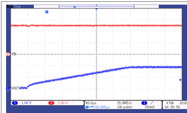
图 7-3. TPS737-Q1 启动
