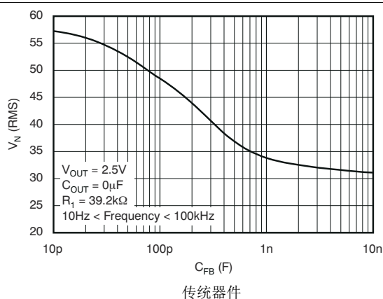
图 5-29. TPS73701-Q1 RMS 噪声电压与 C_{FB} 间的关系
