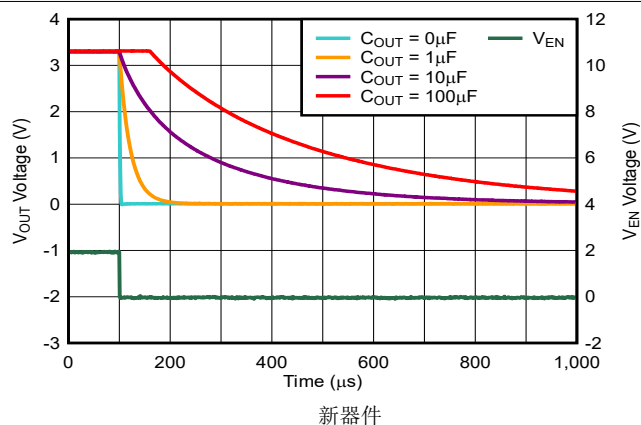
图 5-42. TPS73701-Q1 关断响应
