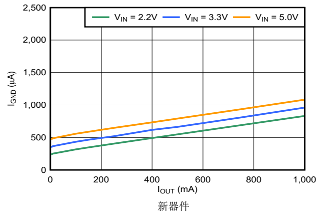
图 5-12. 接地引脚电流与输出电流间的关系
