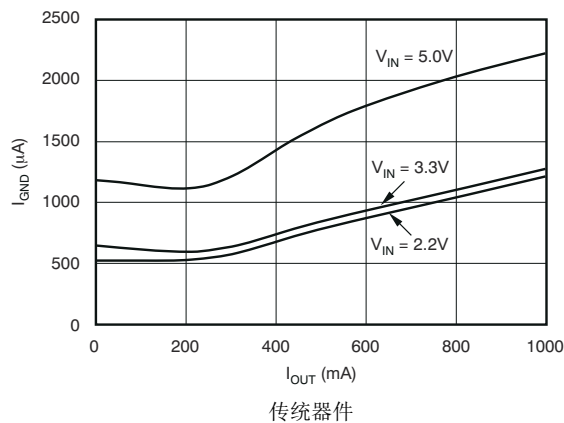
图 5-11. 接地引脚电流与输出电流间的关系
