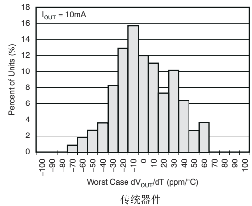
图 5-10. 压降电压漂移柱状图
