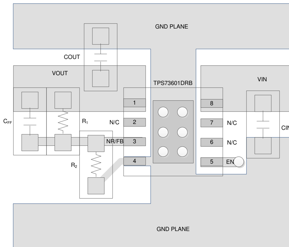
图 7-7. 可调输出电压选项布局 ( DRB 封装 )
