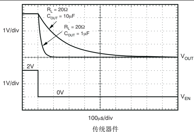
图 5-41. TPS73701-Q1 关断响应
