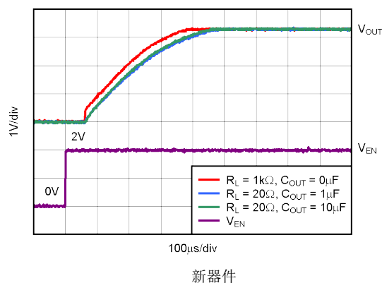
图 5-40. TPS73701-Q1 导通响应
