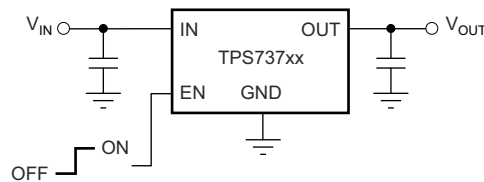
图 7-1. 固定电压版本的典型应用电路
