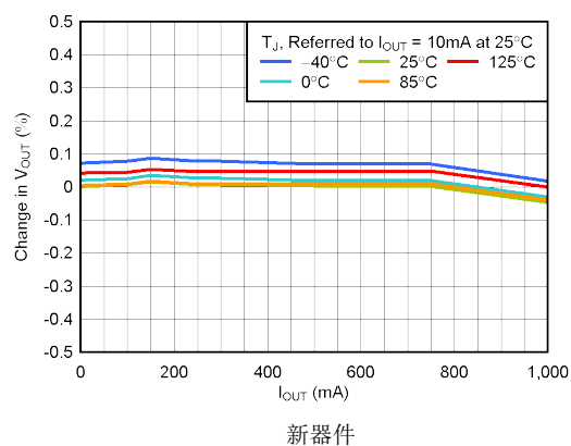
图 5-2. 负载调整率
