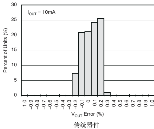
图 5-9. 输出电压柱状图
