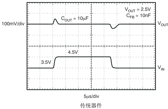
图 5-51. TPS73701-Q1 线路瞬态, 可调节版本
