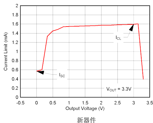
图 5-18. 电流限值与 V_{OUT} (折返) 间的关系
