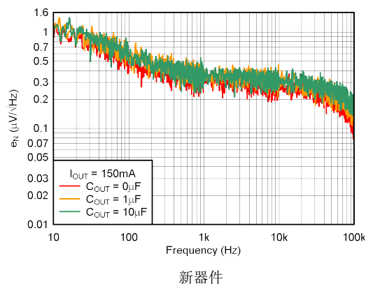
图 5-28. 噪声频谱密度
