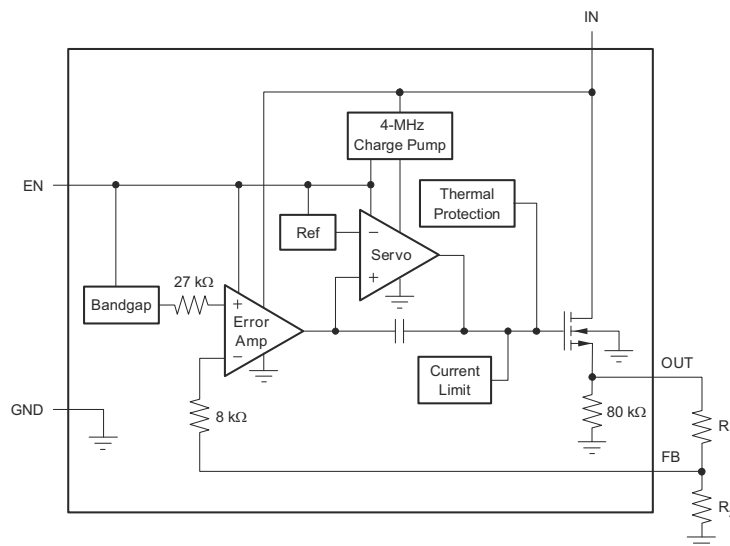
图 6-2. 可调电压版本
