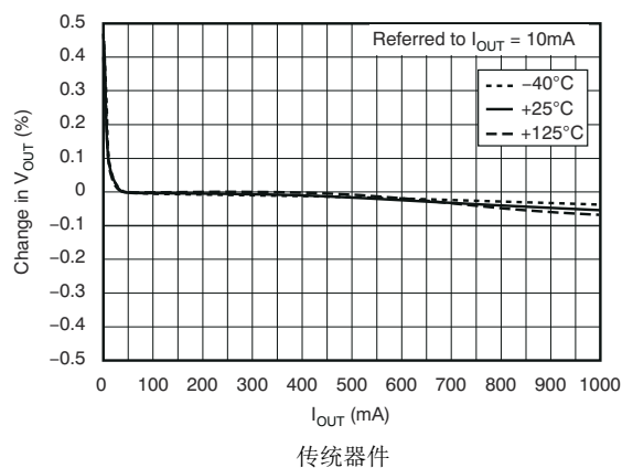
图 5-1. 负载调整率
