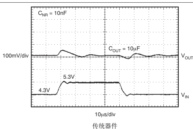
图 5-37. TPS73733-Q1 线路瞬态响应
