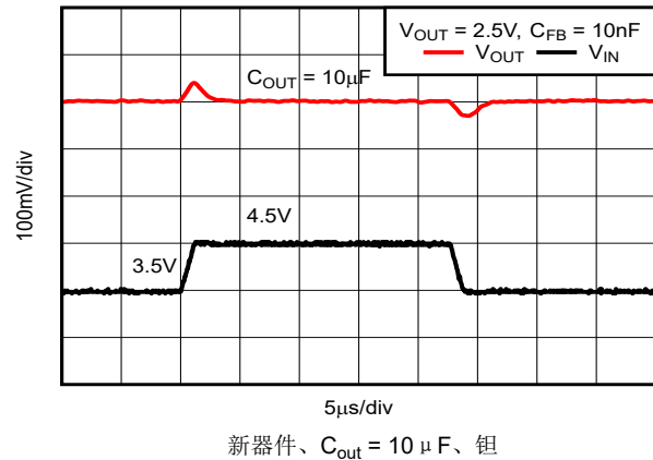
图 5-52. TPS73701-Q1 线路瞬态, 可调节版本
