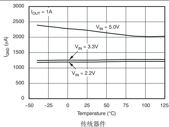
图 5-13. 接地引脚电流与温度间的关系
