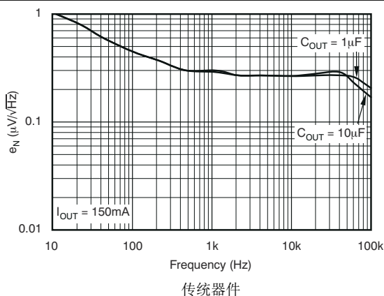
图 5-27. 噪声频谱密度
