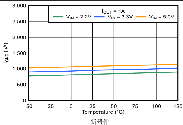
图 5-14. 接地引脚电流与温度间的关系
