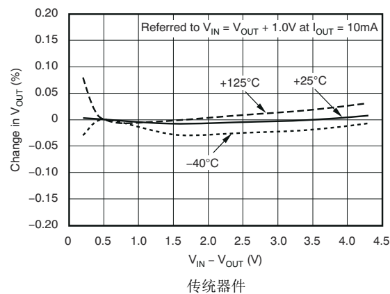
图 5-3. 线性调整率
