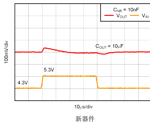
图 5-38. TPS73733-Q1 线路瞬态响应
