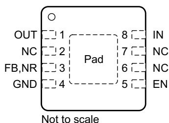
图 4-1. DRB 封装，8 引脚 VSON（顶视图）
