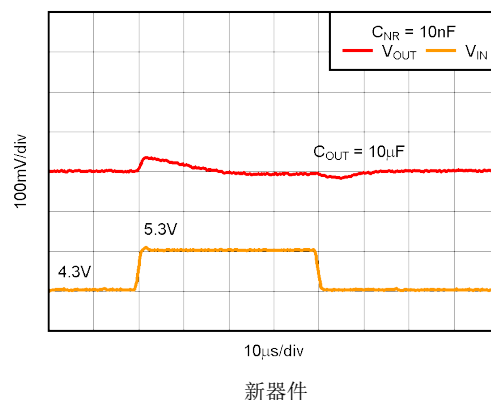
图 5-38. TPS73733 线路瞬态响应
