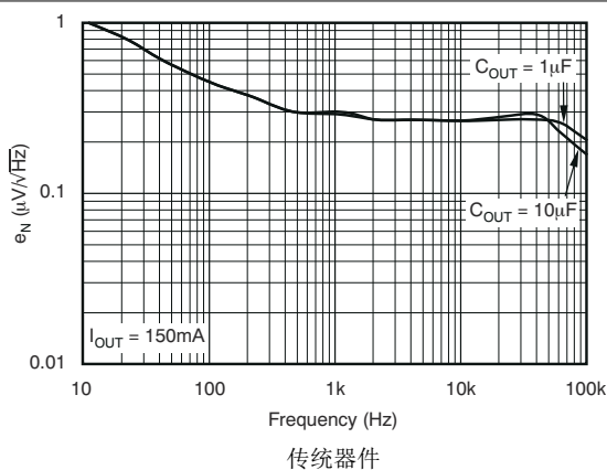
图 5-27. 噪声频谱密度
