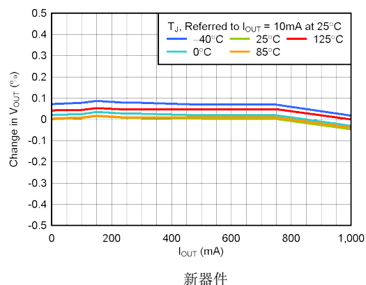
图 5-2. 负载调整率
