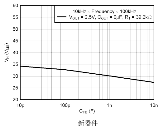
图 5-30. TPS73701 RMS 噪声电压与 C_{FB} 间的关系
