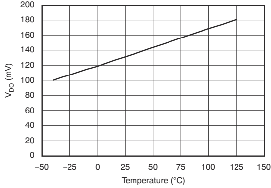
图 5-7. 压降电压与温度间的关系
