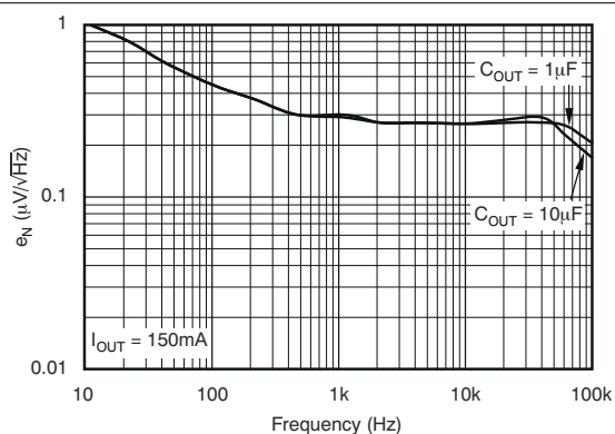
图 7-5. 噪声频谱密度
