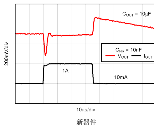
图 5-36. TPS73733 负载瞬态响应
