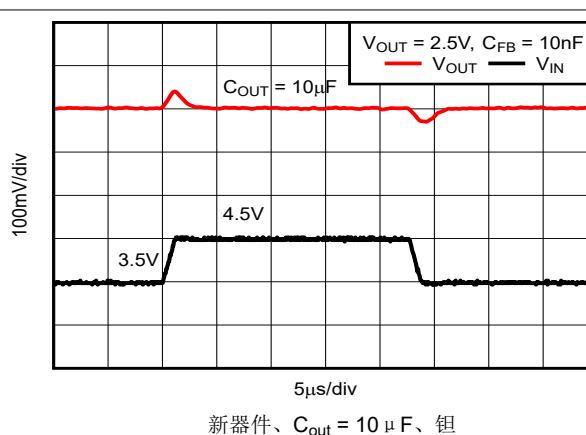
图 5-52. TPS73701 线路瞬态, 可调节版本
