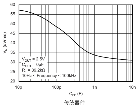
图 5-29. TPS73701 RMS 噪声电压与 C_{FB} 间的关系
