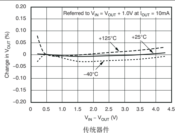
图 5-3. 线性调整率
