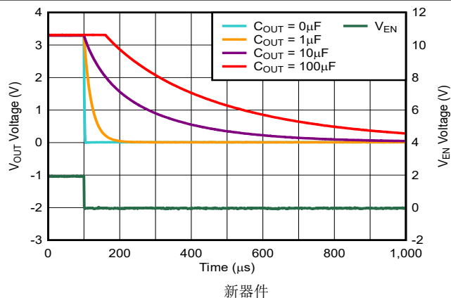
图 5-42. TPS73701 关断响应
