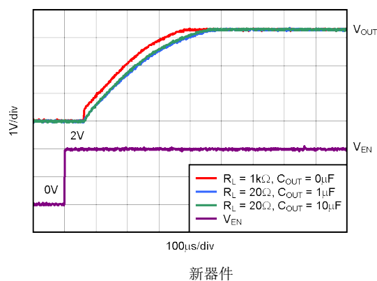
图 5-40. TPS73701 导通响应
