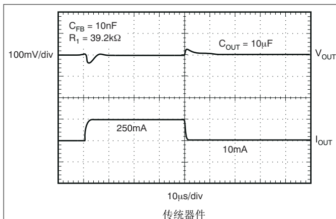
图 5-49. TPS73701 负载瞬态, 可调节版本
