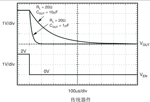
图 5-41. TPS73701 关断响应
