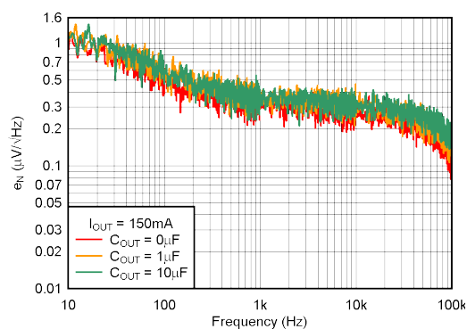
图 7-6. 噪声频谱密度
