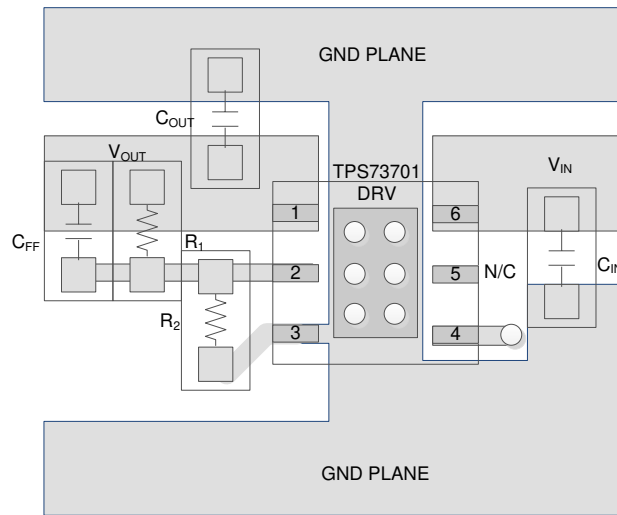
图 7-12. 布局示例
