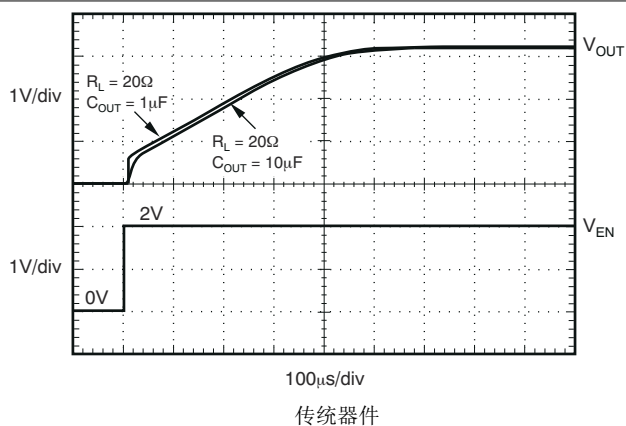
图 5-39. TPS73701 导通响应
