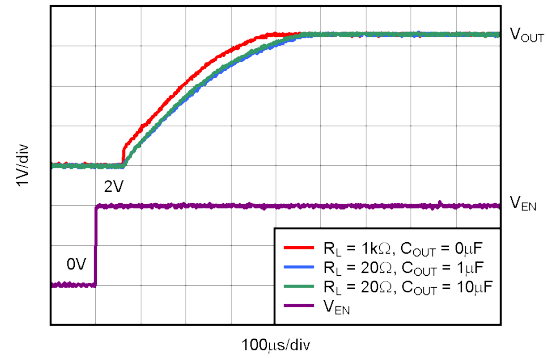
图 7-4. TPS73633 Turn-On Response
