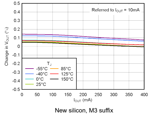
图 5-2. Load Regulation
