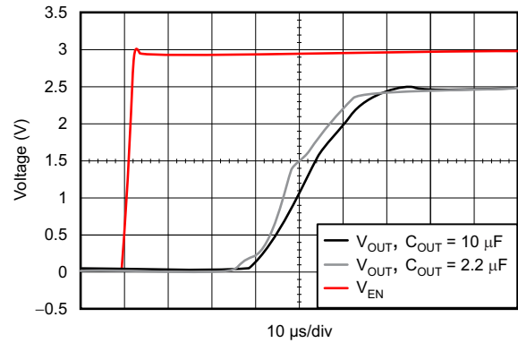
图 18. TPS735 Turnon Response Using EN
