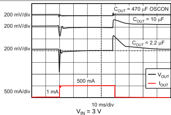
图 20. TPS735 Load Transient Response
