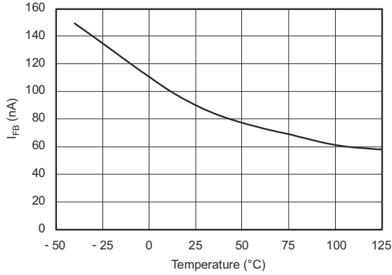
图 5-49. TPS73201-Q1 - I_{FB} 与温度间的关系
