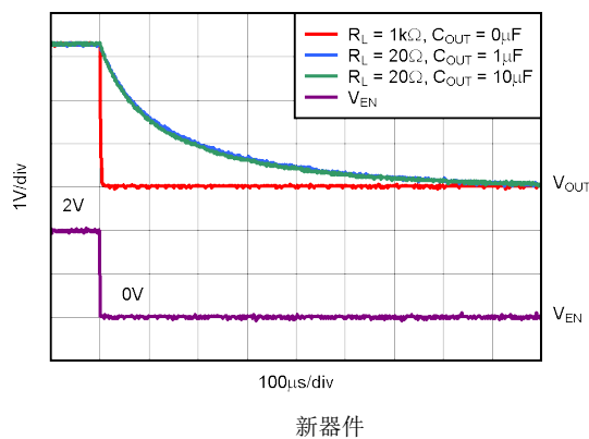
图 5-42. TPS73233-Q1 关断响应
