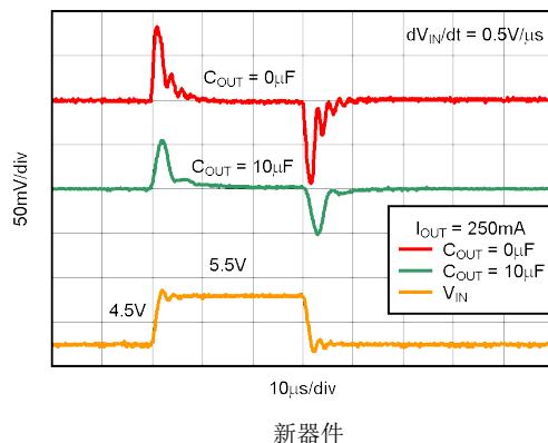
图 5-38. TPS73233-Q1 线路瞬态响应
