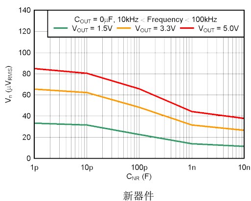
图 5-34. RMS 噪声电压与 C_{NR} 间的关系
