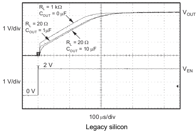
图 5-39. TPS73233 Turn-On Response
