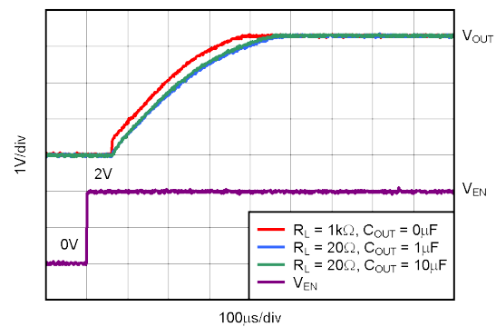
图 5-40. TPS73233 Turn-On Response
