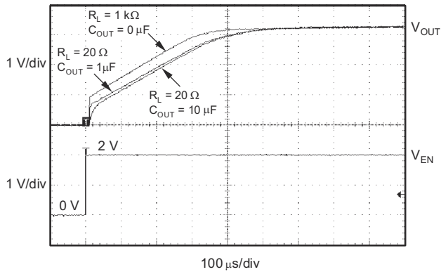
图 7-3. TPS73233 Turn-On Response
