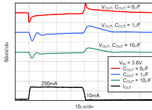
图 7-6. TPS73233 Load Transient Response
