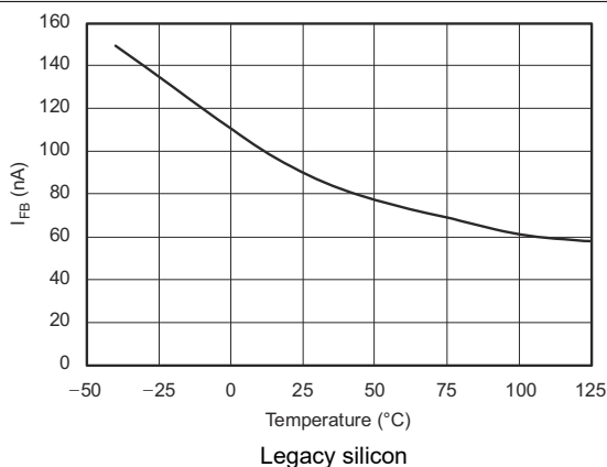
图 5-49. TPS73201 I_{FB} vs Temperature
