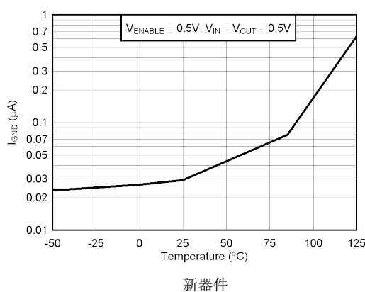
图 5-16. 关断时的接地引脚电流与温度间的关系
