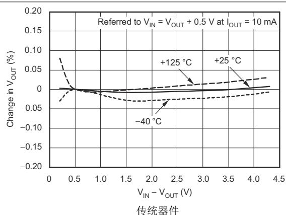
图 5-3. 线路调整
