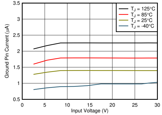
图 5-14. 1.2V 接地引脚电流与 V_{\text{IN}} 和温度间的关系
