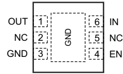
图 4-2. DRV 封装，WSO6-6 (顶视图)
