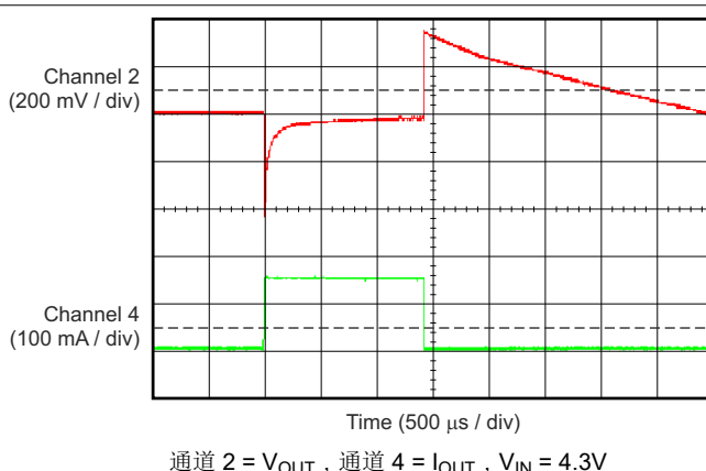
图 5-32. TPS70933-Q1 负载瞬态 (1mA 至 150mA)
