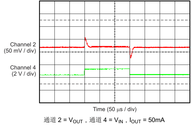
图 5-38. TPS70933-Q1 线路瞬态 (4.3V 至 5.3V)
