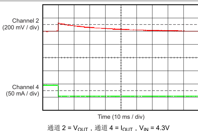
图 5-33. TPS70933-Q1 负载瞬态 (50mA 至 0mA)
