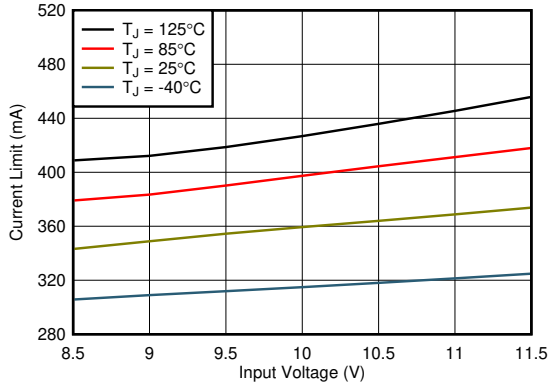
图 5-13. 6.5V 电流限制与 V_{\text{IN}} 和温度间的关系
