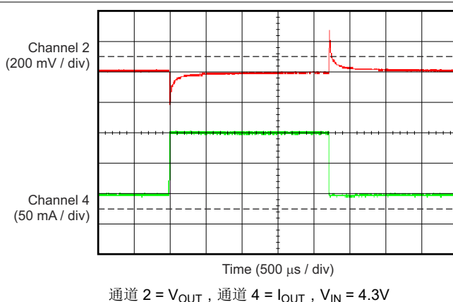
图 5-34. TPS70933-Q1 负载瞬态 (50mA 至 150mA)
