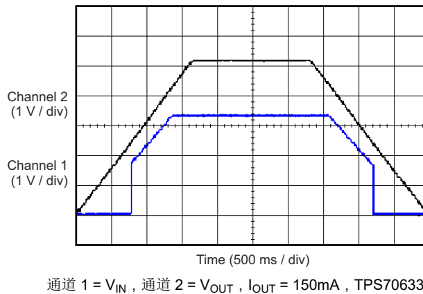
图 5-41. 上电和下电响应
