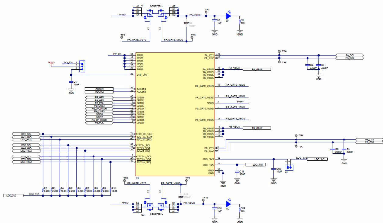
图 11-1. Example Schematic
