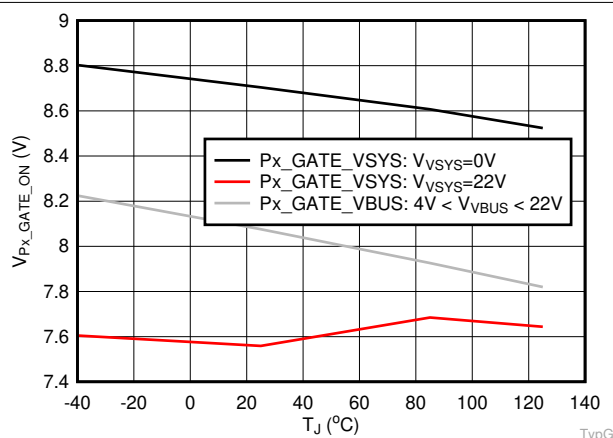
图 6-5. V Px_GATE_ON vs. Temperature
