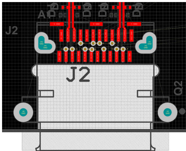
图 11-7. Type-C Connector SSTXRX Top Layer
