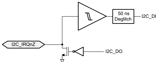
图 9-51. IOBUF_I2C I/O
