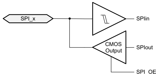
图 9-52. IOBUF_GPIOHSSPI
