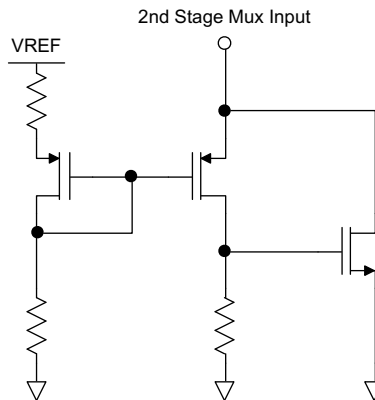
图 9-37. Port Mux Clamp
