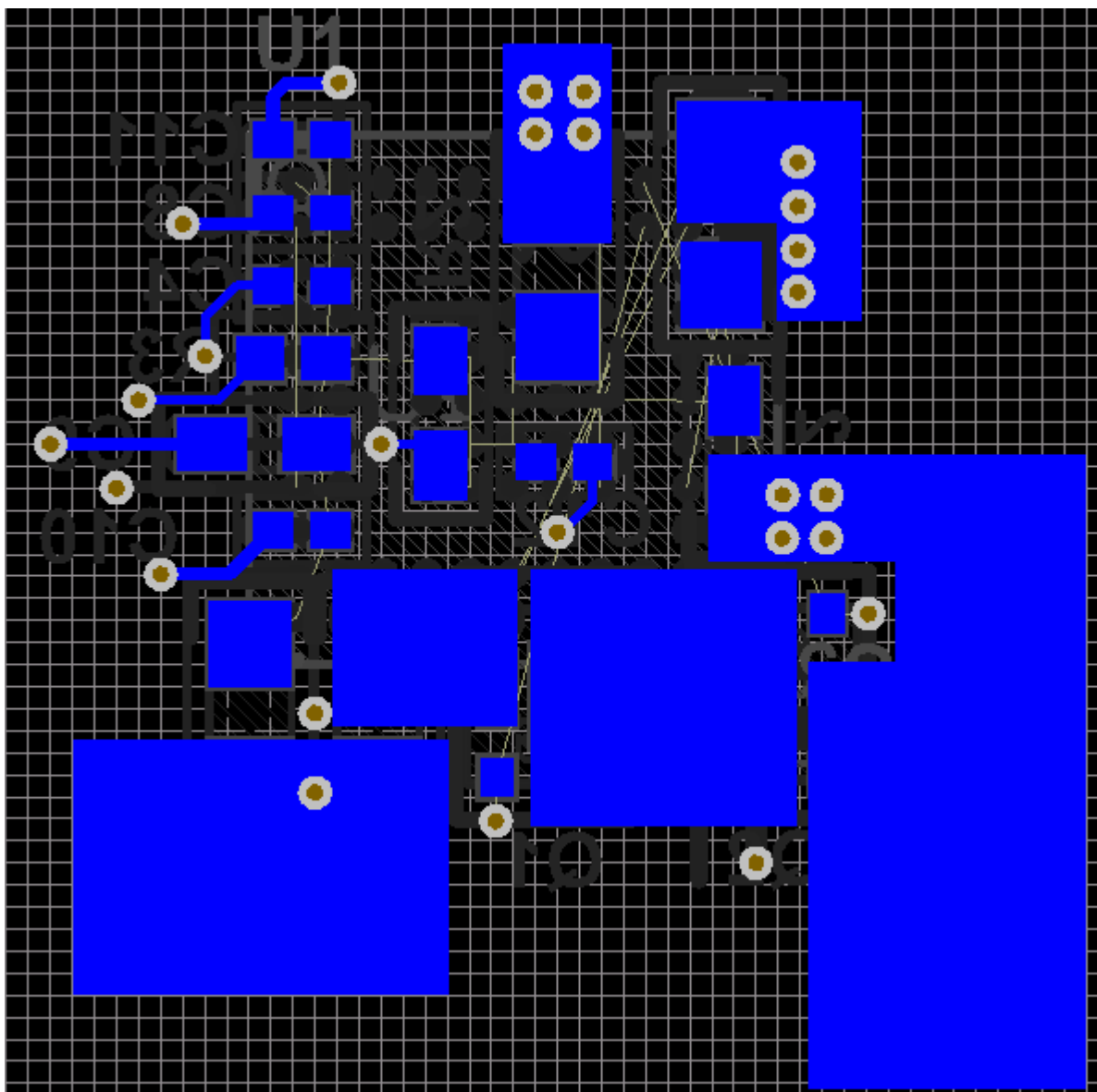
图 12-14. Bottom Layer Component Routing
