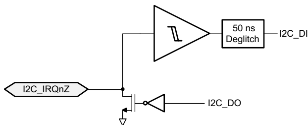
图 9-51. IOBUF_I2C I/O
