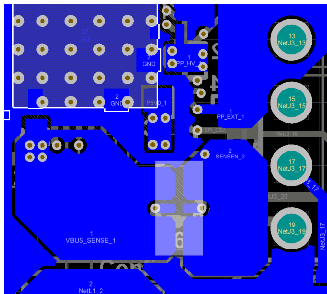
图 12-8. Bottom Polygonal Pours
