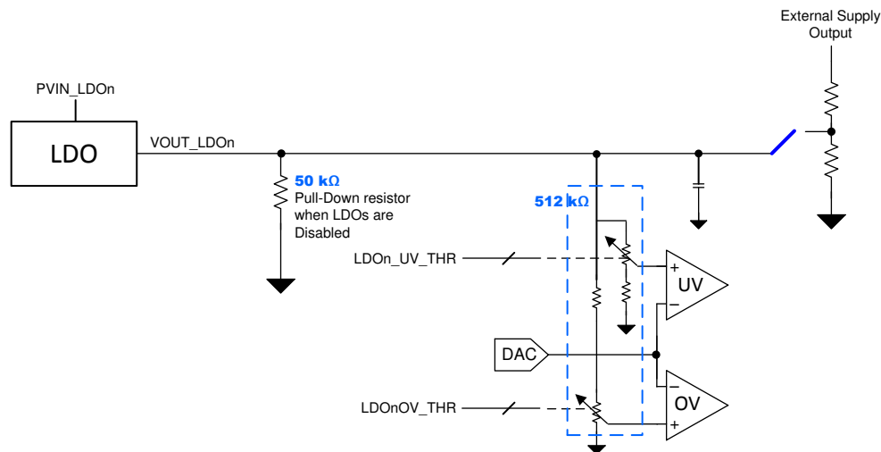
图 8-9. Impedance at the VOUT_LDO Pins
