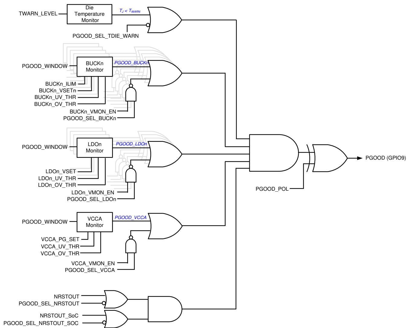
图 8-11. PGOOD Block Diagram
