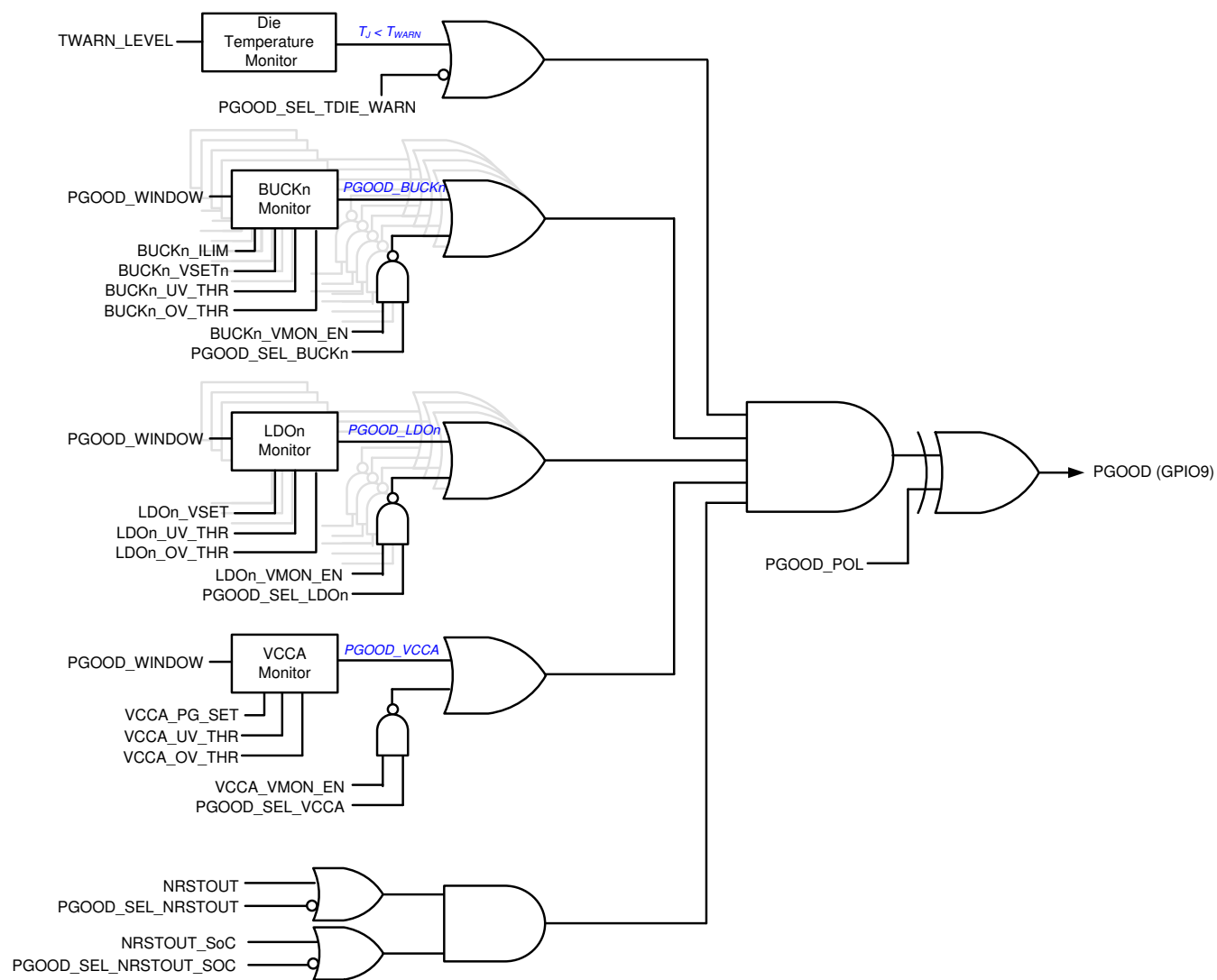
图 8-10. PGOOD Block Diagram
