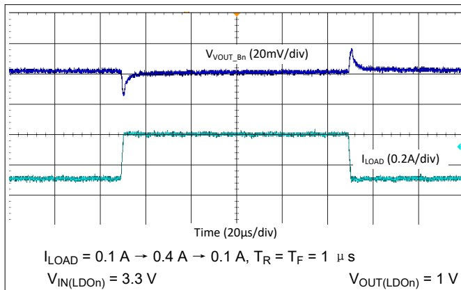
图 9-64. LDO1/2/3 Load Step Transient
