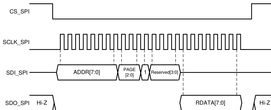
图 8-60. SPI Read Cycle
