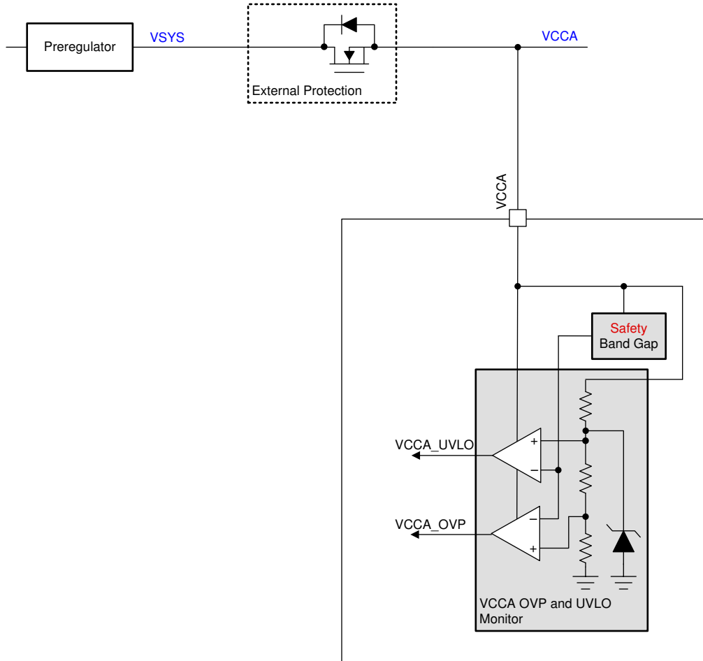
图 8-1. VCCA Monitor
