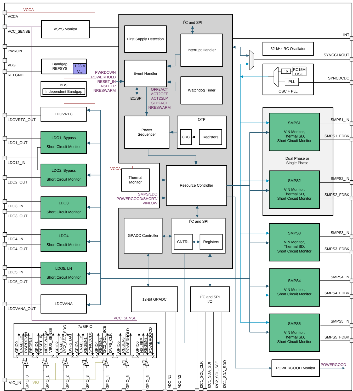
图 1-1. 功能图
