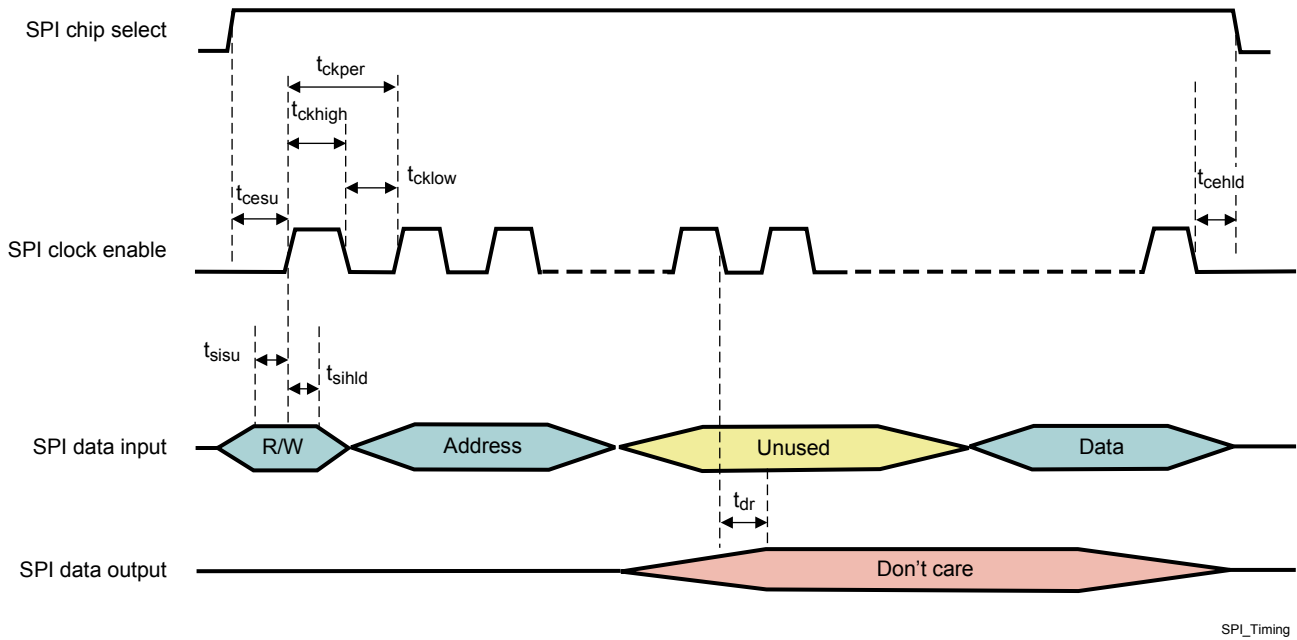
图 5-3. SPI Interface Timing Diagram
