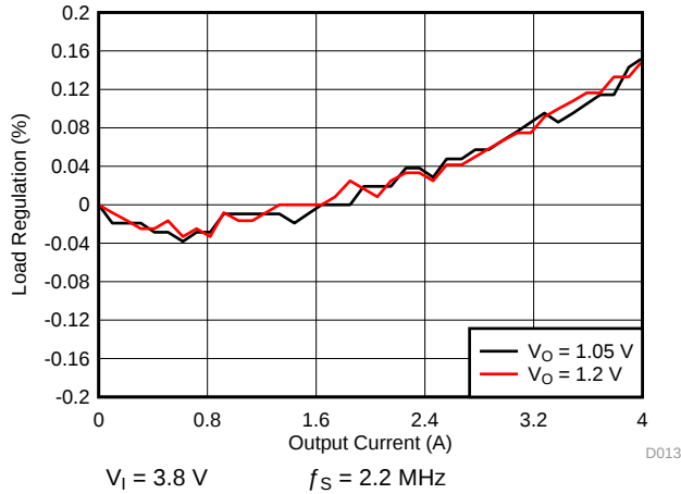
图 7-9. SMPS Load Regulation for 4-A Dual Phase
