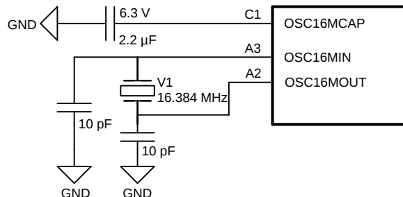
图 7-6. Crystal Input Configuration
