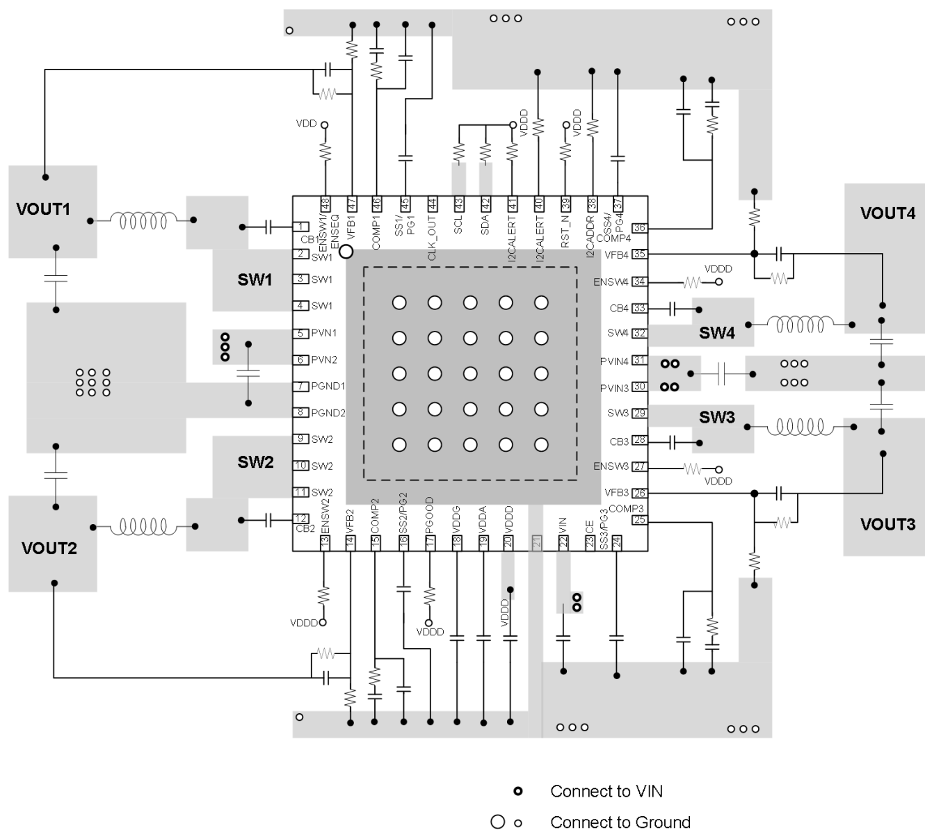
图 11-1. Layout Schematic
