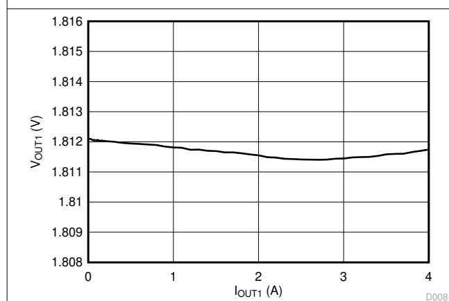
图 9-7. V_{OUT1} Load Regulation
