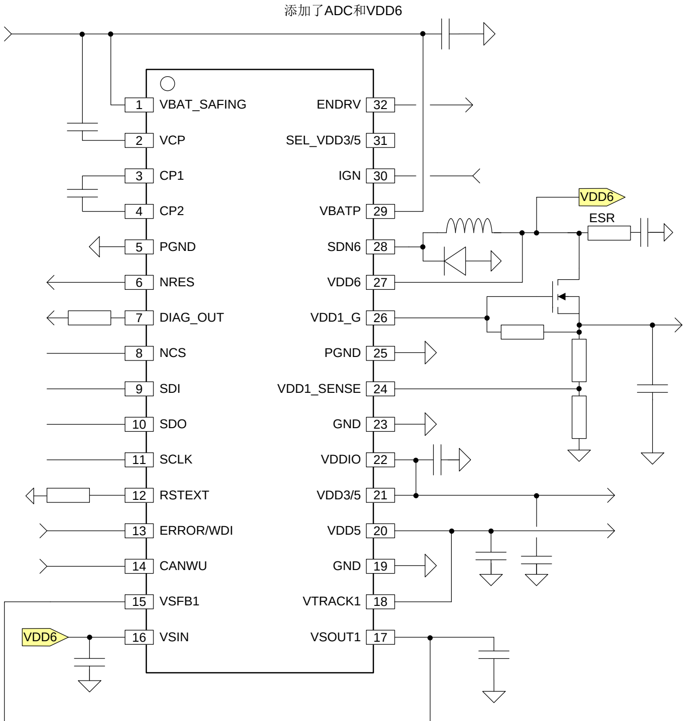
图 1-1. 典型应用图
