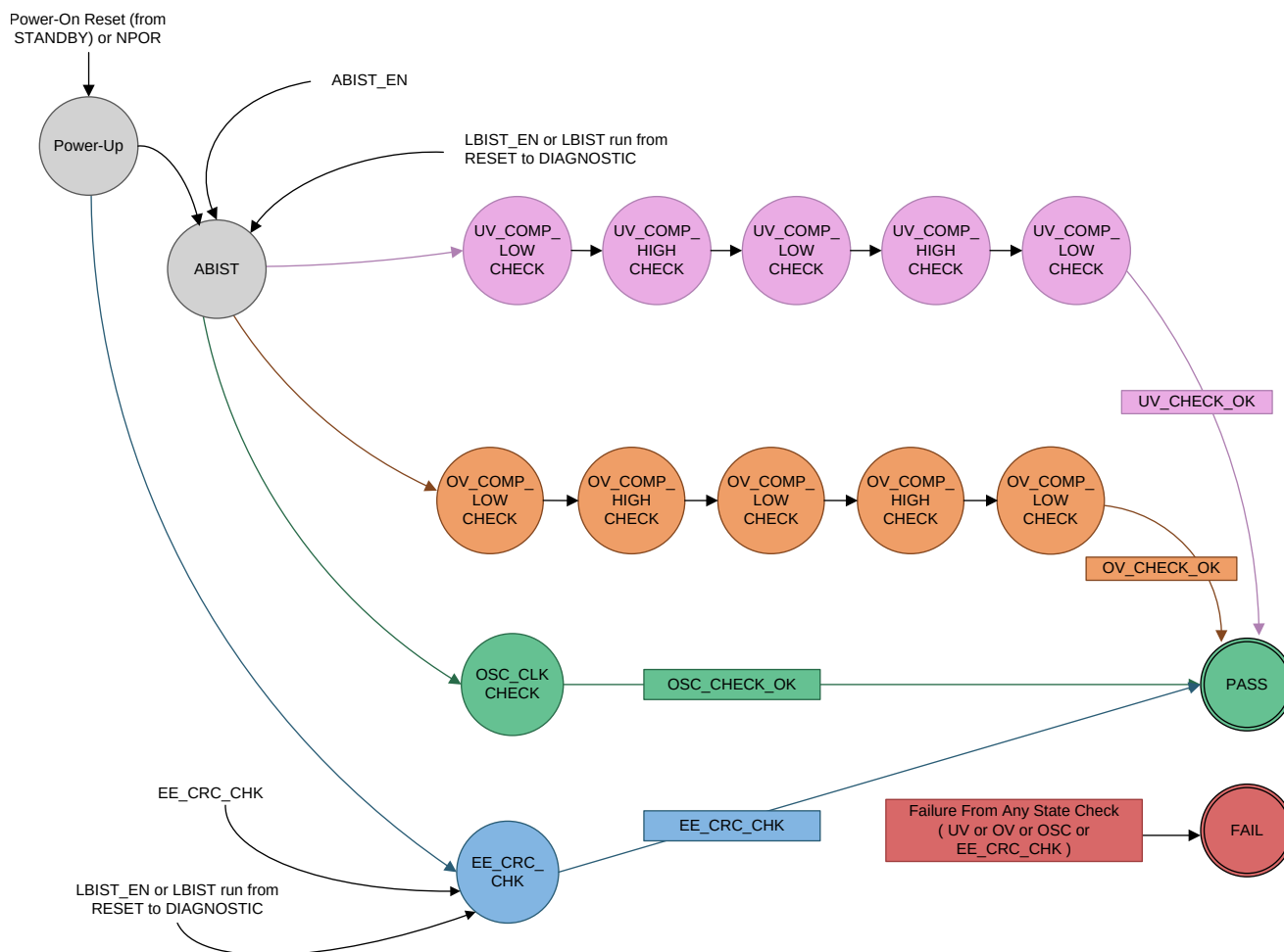
Figure 5-3. 模拟 BIST 运行状态
