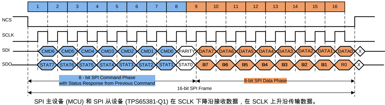
Figure 5-17. 16 位 SPI 帧
