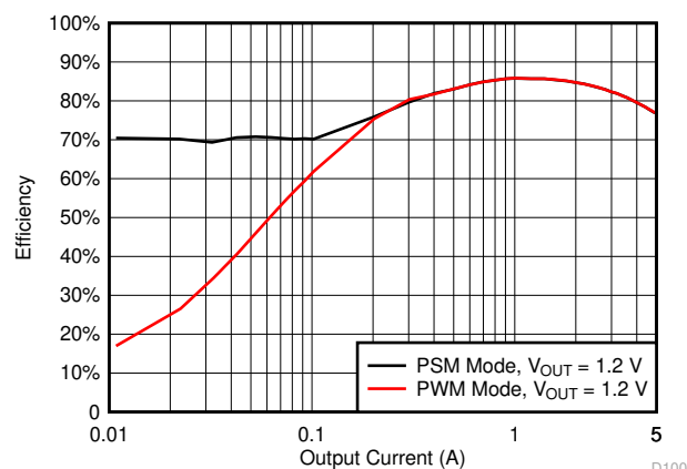
效率与输出负载之间的关系
