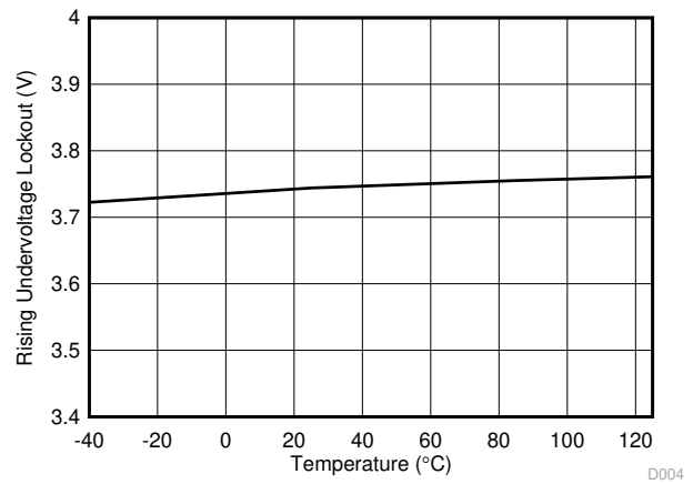
图 7-4. Vin UVLO Raising vs Temperature
