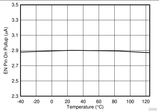
图 7-6. EN Pin Pullup Current vs Temperature, EN = 1.0 V
