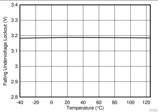
图 7-5. Vin UVLO Falling vs Temperature
