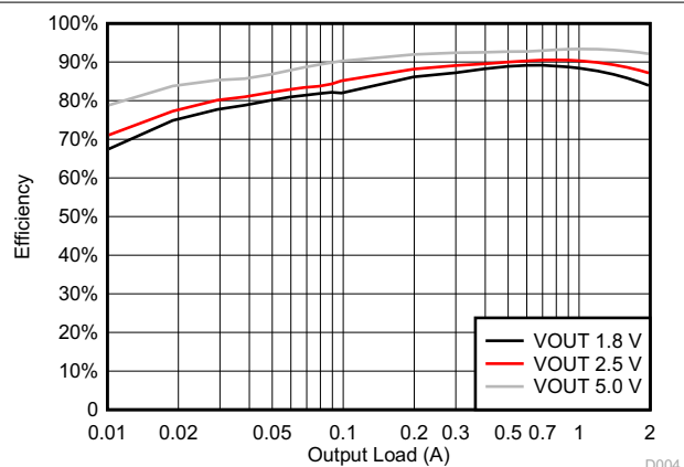
图 6-3. BUCK3 Efficiency
