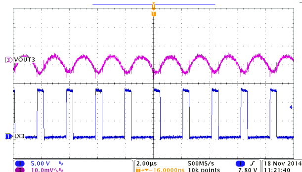
A. Iout = 3 A 图 8-6. BUCK1, Output Voltage Ripple
