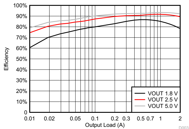
图 6-2. BUCK2 Efficiency
