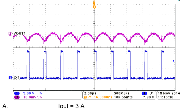
A. Iout = 3 A 图 8-6. BUCK1, Output Voltage Ripple
