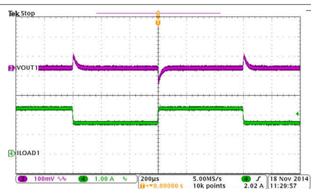
图 8-10. BUCK1, Load Transient
