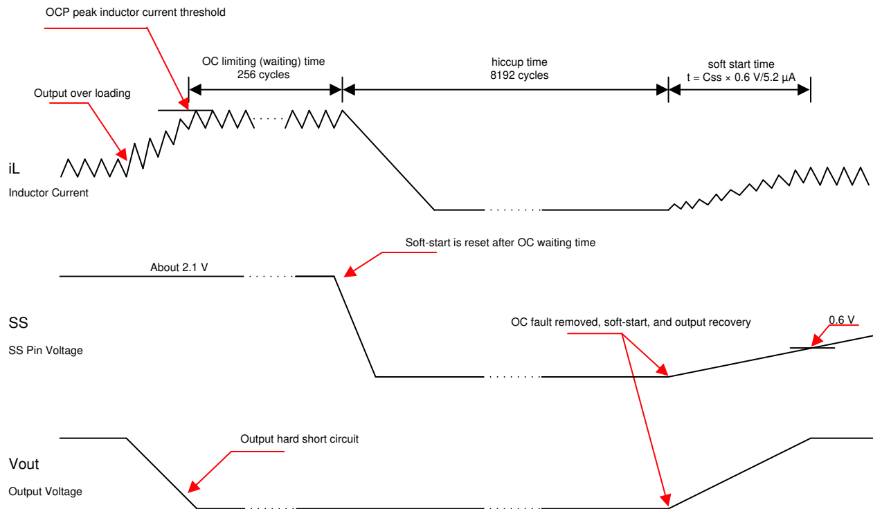
图 7-11. Overcurrent Protection
