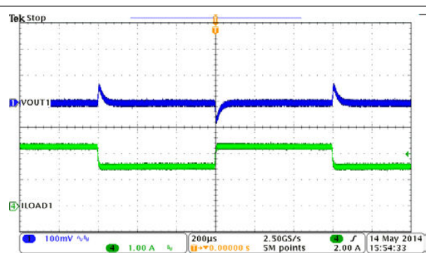
图 9-9. BUCK1, Load Transient, 1.5 to 2.25 A SR = 0.25 A/µs
