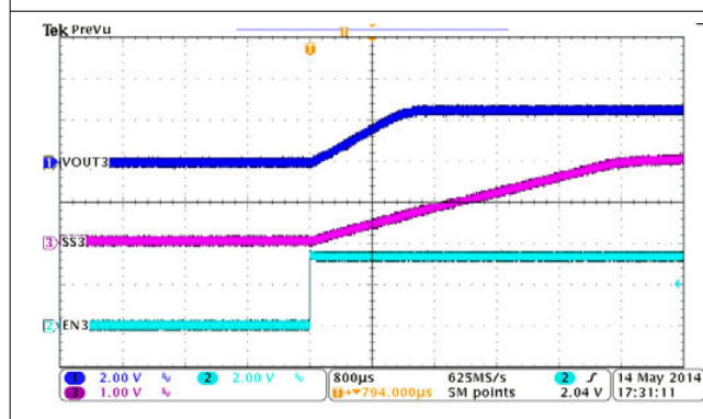
图 9-4. BUCK3, Soft-Start, Iout = 2 A
