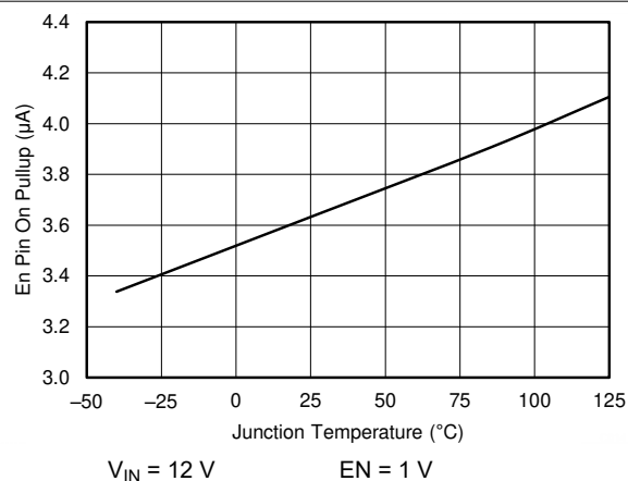
图 6-12. EN Pin Pull-Up Current vs Temperature, EN=1.0V
