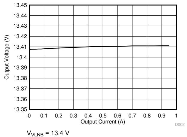
图 6-2. Load Regulation
