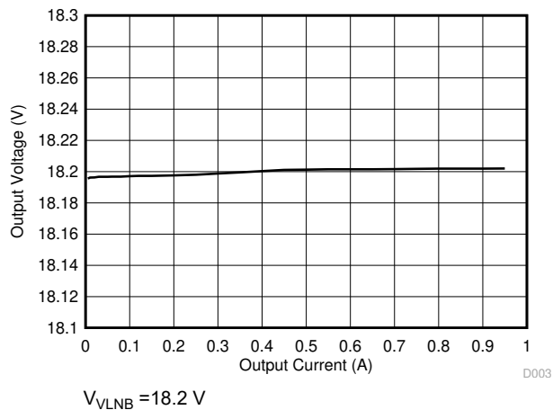
图 6-3. Load Regulation
