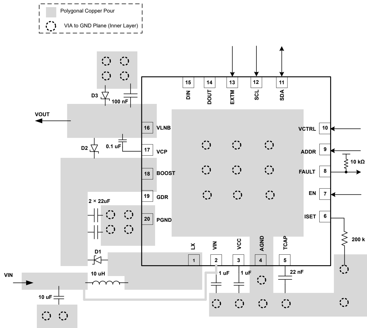
图 8-22. Layout
