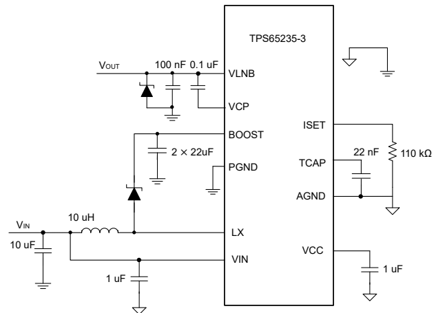
简化原理图
