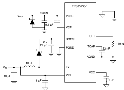
简化原理图
