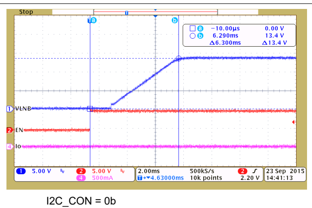
图 7-4. VLNB Output Controlled by EN Pin
