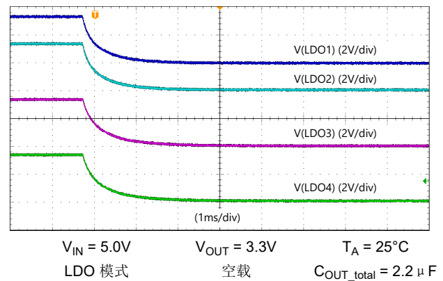
图 7-9. LDO 放电
