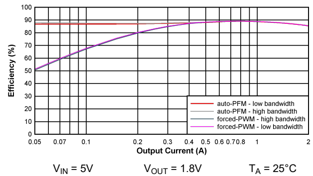
图 5-2. BUCK23 效率
