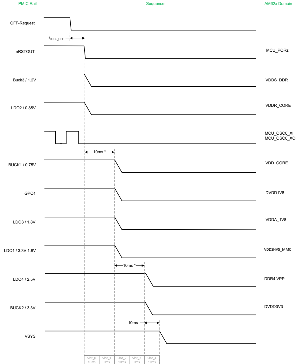
图 7-3. 断电时序 (示例)
