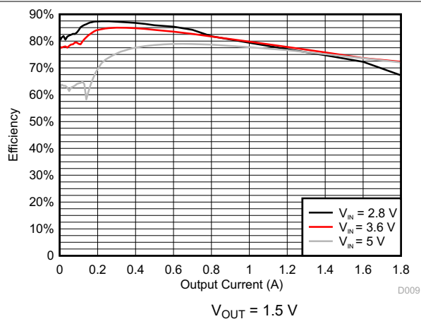
图 8-6. DCDC3 Efficiency
