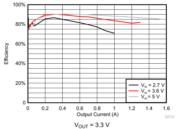
图 9-7. DCDC4 Efficiency
