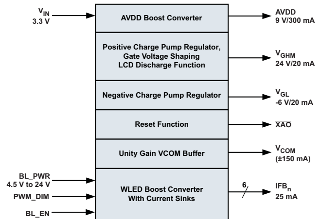
简化框图
