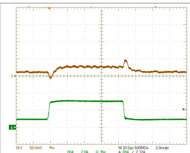
图 8-5. BUCK3 Converter Load Transient
