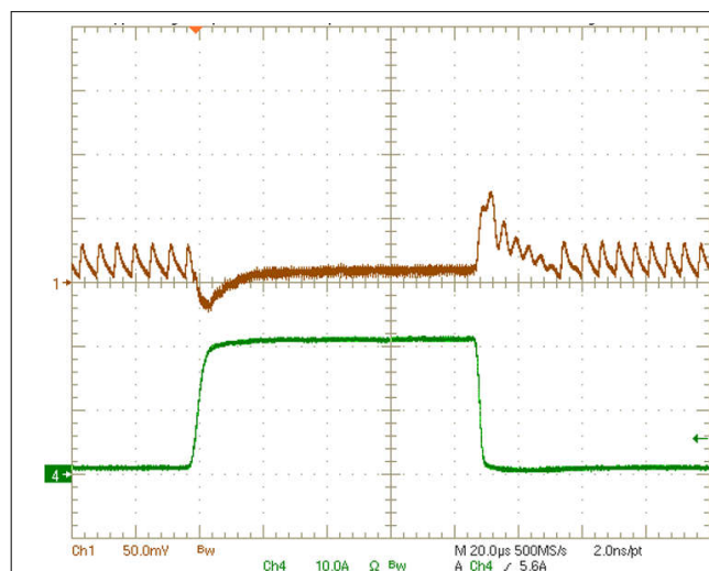
图 8-4. BUCK2 Controller Load Transient
