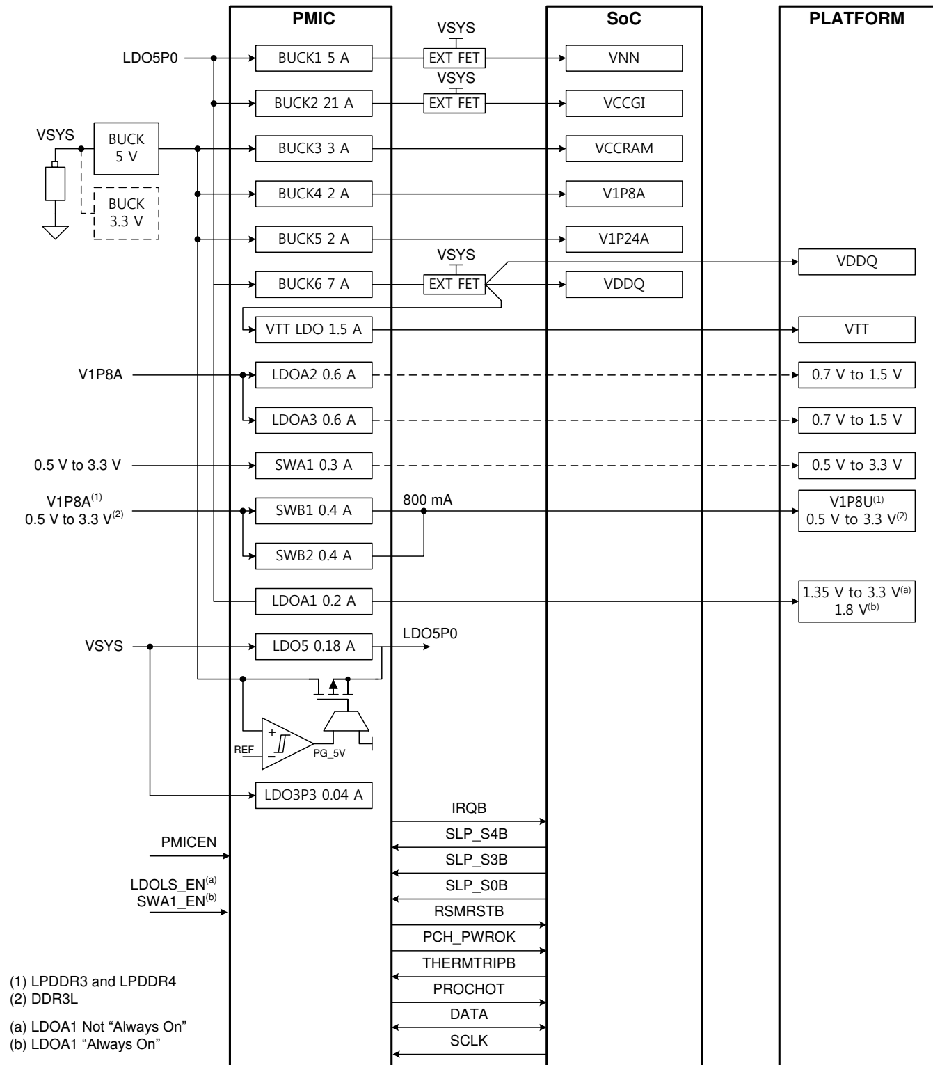
图 7-2. Apollo Lake Power Map
