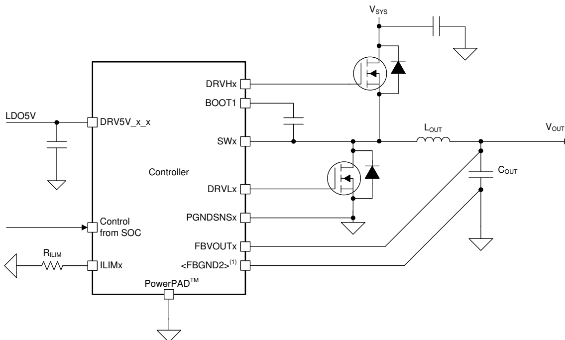
图 7-3. Controller Diagram
