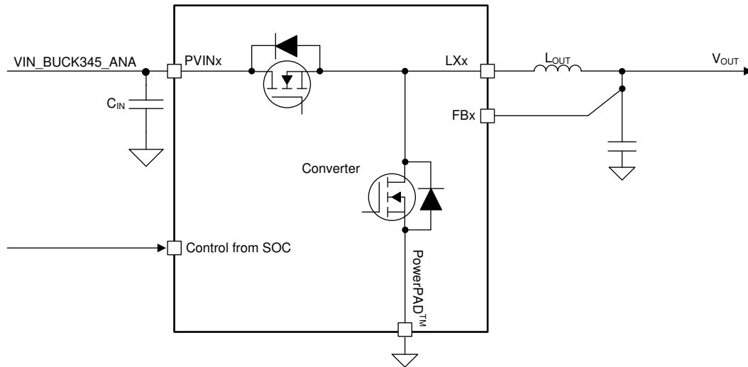
图 7-3. Converter Diagram
