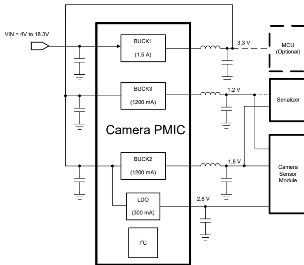
TPS650350-Q1 应用电路
