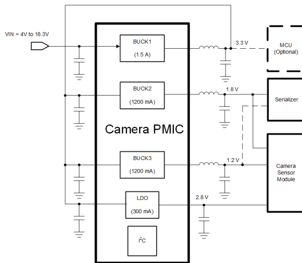
TPS650333-Q1 应用电路
