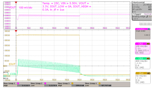
图 8-27. Load Transient, 300 mA Step
