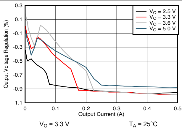
图 8-18. Load Regulation
