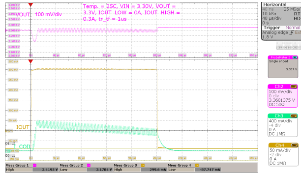
图 8-26. Load Transient, 300 mA Step
