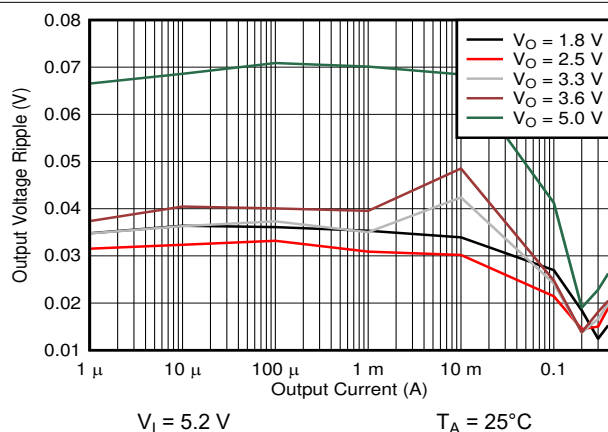
图 8-16. Output Voltage Ripple
