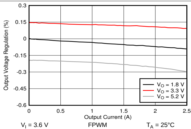
图 34. Load Regulation
